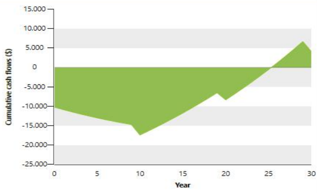
Gambar 8: Grafik nilai investasi dengan penggantian baterai
