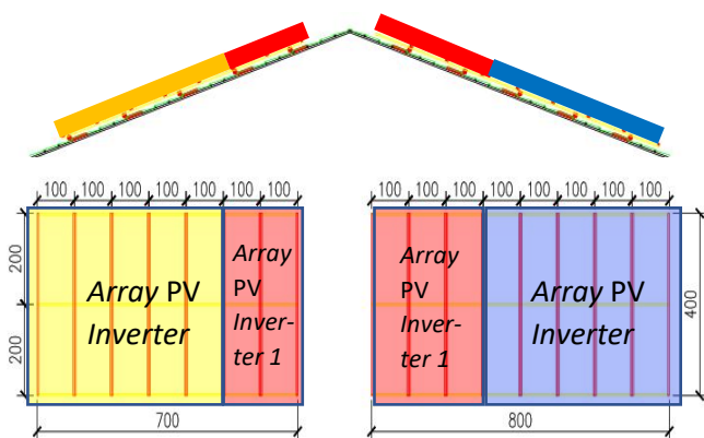
Gambar 2: Posisi Masing-masing Array PV pada Atap Gedung Kantor
