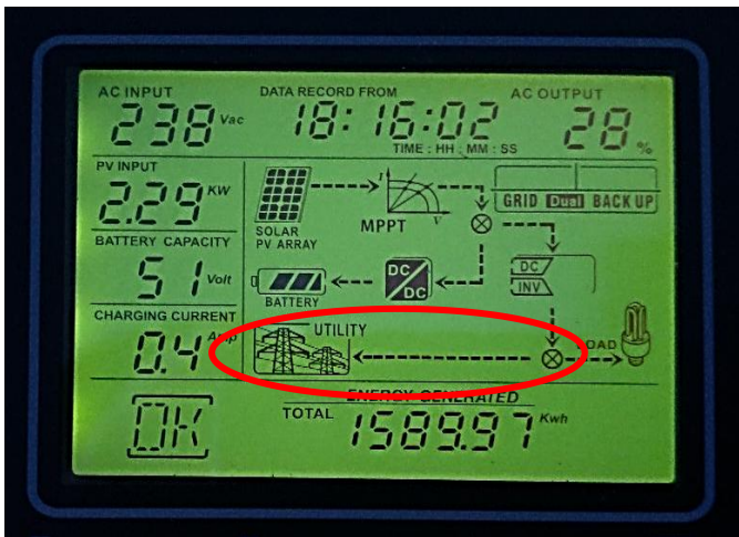
Gambar 6: Tampilan/ Display Salah Satu Inverter
