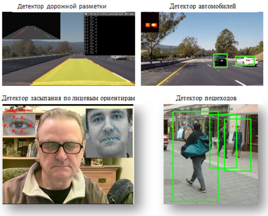
Рис. 2. Примеры работы некоторых программных модулей компьютерного зрения для подключенных автомобилей (выполнено автором).
