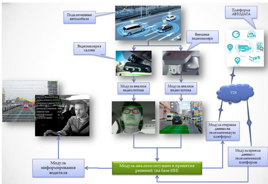
Рис. 1. Принципиальная схема работы программных средств компьютерного зрения для подключенных автомобилей (выполнено автором).
