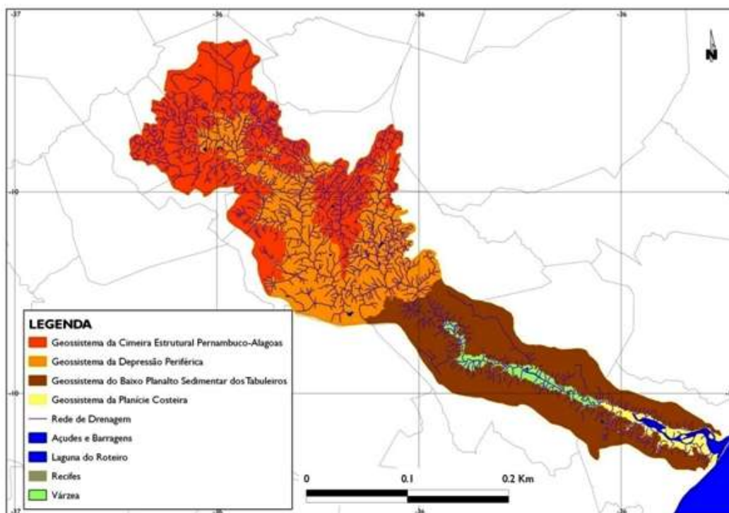
Figura 04: Geossistemas da bacia do rio São Miguel.
