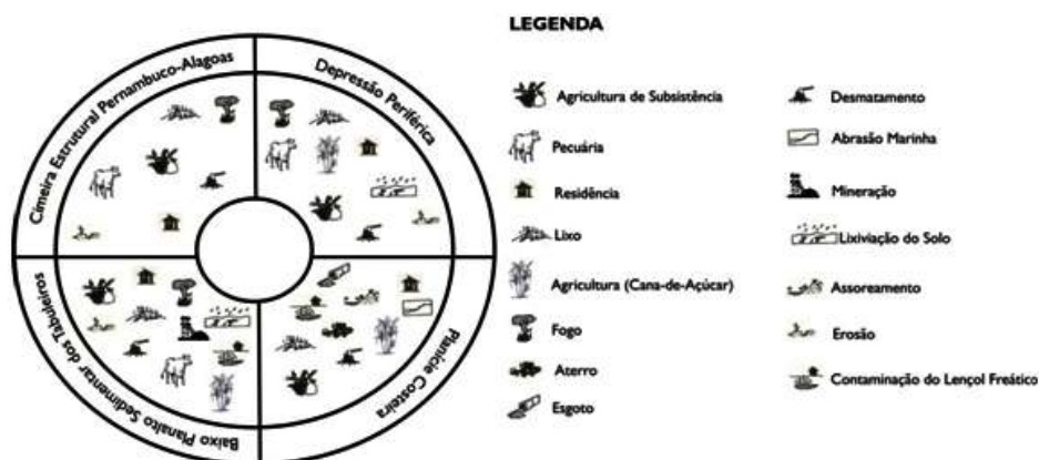
Figura 05: Principais Impactos Ambientais nos Geossistemas da Bacia do Rio São Miguel Fonte: Adaptado de Vicente da Silva (1998, apud RODRIGUEZ et al, 2007), por Souza, 2012.
