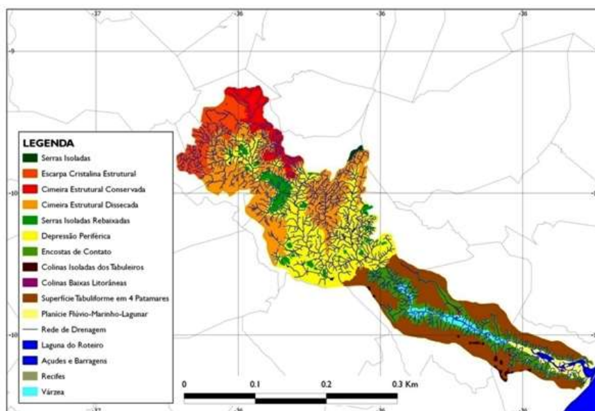
Figura 03: Compartimentação geomorfológica da bacia do rio São Miguel. Fonte: SOUZA, 2013.
