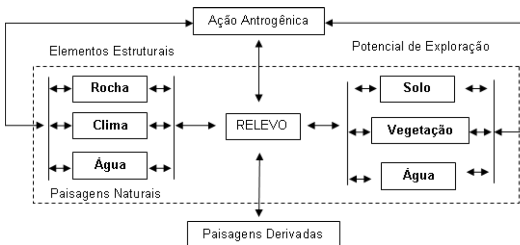
Figura 01. O relevo é principal elemento integrante da paisagem. Fonte: SOBRINHO FALCÃO, 2007 (adaptado pelo autor)
