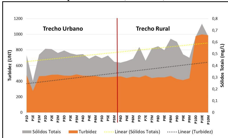
Figura 4 – Comportamento da concentração de Turbidez e Sólidos Totais no rio Acre – período de cheia (21/fev/2019)
