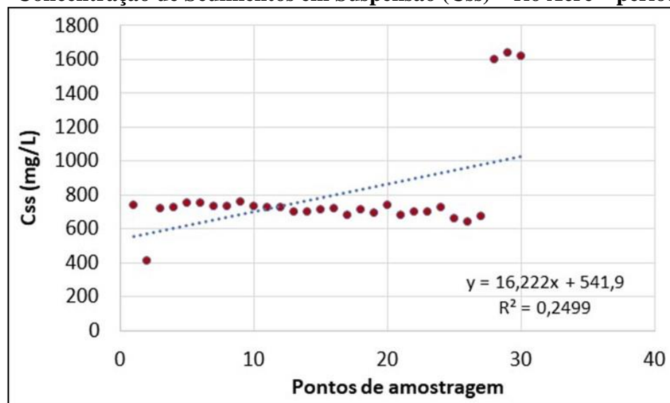
Figura 5 – Concentração de Sedimentos em Suspensão (C ss ) – rio Acre – período de cheia
