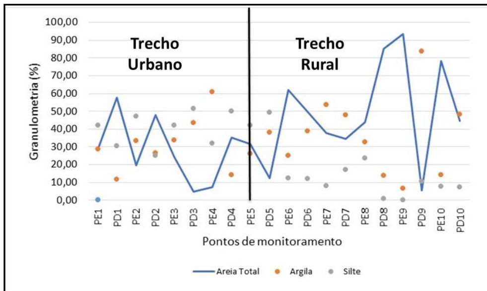
Figura 4 - Análise granulométrica dos sedimentos de fundo do médio rio Acre
