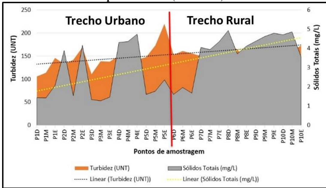
Figura 2 – Comportamento da concentração de Turbidez e Sólidos Totais no rio Acre – período de seca (20/set/2018)
