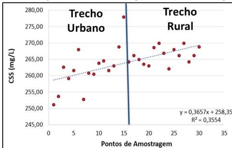
Figura 3 – Concentração de Sedimentos em Suspensão (C ss ) – rio Acre – período seco
