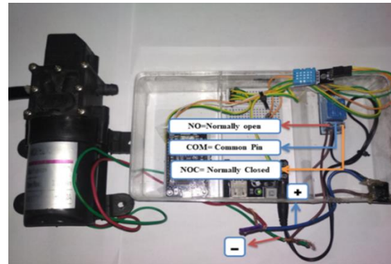
Gambar 5. Perakitan Alat
