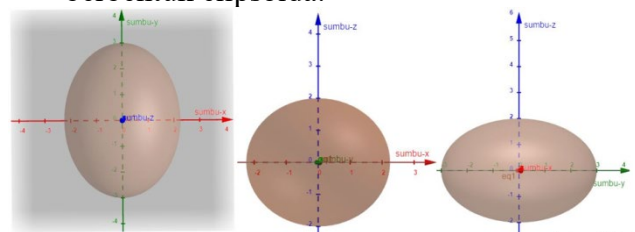
Gambar 4.2 Benda permukaan kuadratis pada bidang x dan y, bidang x dan z serta bidang y dan z
