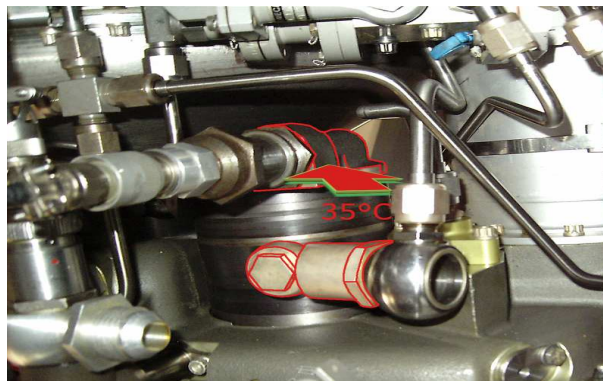
FIG. 6: Vue augmentée de l'opérateur après un "Outlining". L'expert a sélectionné les éléments d'intérêt et indiqué la température d'un objet.
