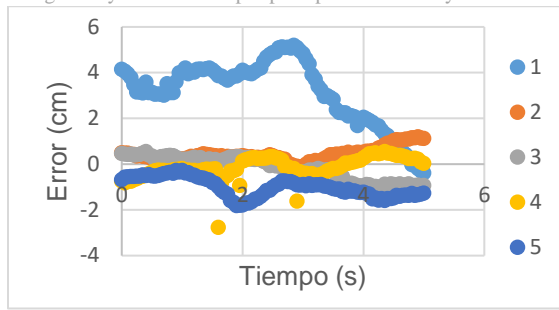
Figura 37: Error absoluto de los valores en Y del brazo izquierdo. Fuente: Elaboración propia.
