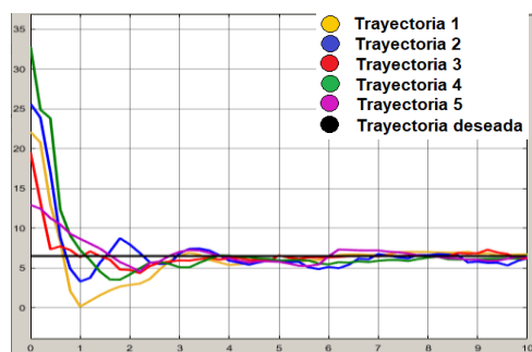
Figura 17: Perfil en X de las 5 trayectorias del brazo derecho. Fuente: Elaboración propia.
