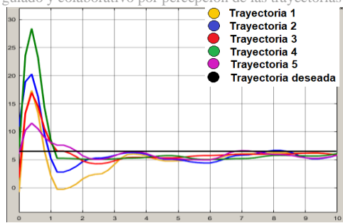
Figura 18: Perfil en X de las 5 trayectorias del brazo derecho con control. Fuente: Elaboración propia.
