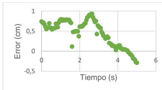
Figura 50: Error promedio de los valores en Y del brazo izquierdo. Fuente: Elaboración propia.
