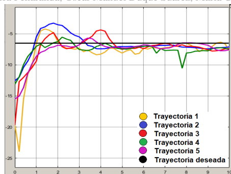
Figura 23: Perfil en x de las 5 trayectorias del brazo izquierdo. Fuente: Elaboración propia.
