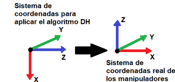
Figura 13: Sistema de coordenadas. Fuente: Elaboración propia.
