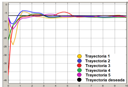
Figura 24: Perfil en X de las 5 trayectorias del brazo izquierdo con control. Fuente: Elaboración propia.
