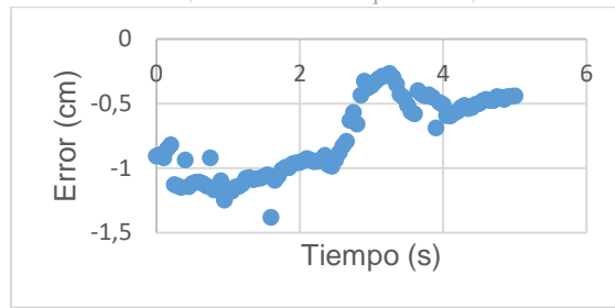
Figura 52: Error promedio de los valores en Z del brazo izquierdo. Fuente: Elaboración propia.
