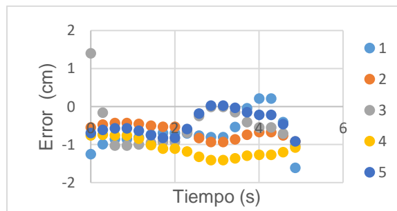
Figura 36: Error absoluto de los valores en X del brazo izquierdo con control. Fuente: Elaboración propia.
