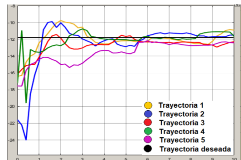
Figura 21: Perfil en Z de las 5 trayectorias del brazo derecho. Fuente: Elaboración propia.
