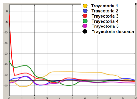
Figura 26: Perfil en Y de las 5 trayectorias del brazo izquierdo con control. Fuente: Elaboración propia.
