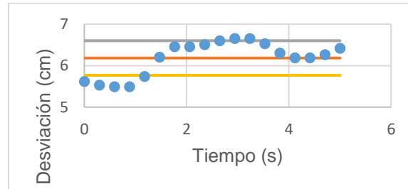
Figura 53: Desviación estándar de los valores en X del brazo derecho con control. Fuente: Elaboración propia.
