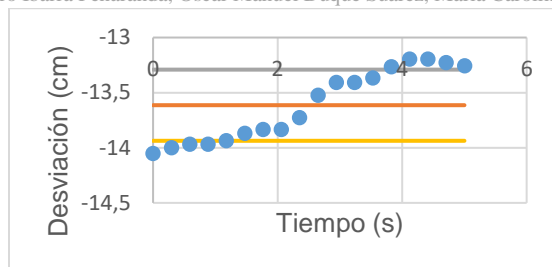
Figura 63: Desviación estándar de los valores en Z del brazo izquierdo con control. Fuente: Elaboración propia.
