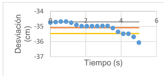
Figura 61: Desviación estándar en Y del brazo izquierdo con control. Fuente: Elaboración propia.
