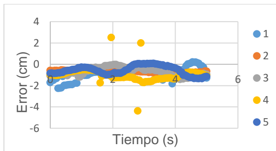
Figura 35: Error absoluto de los valores en X del brazo izquierdo. Fuente: Elaboración propia.
