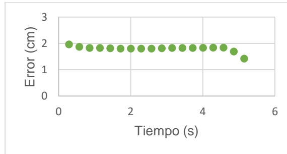
Figura 43: Error promedio de los valores en Y del brazo derecho con control. Fuente: Elaboración propia.
