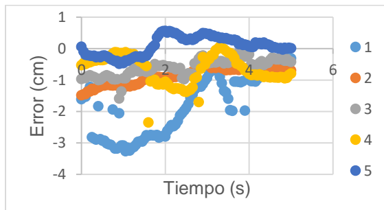
Figura 39: Error absoluto de los valores en Z del brazo izquierdo. Fuente: Elaboración propia.
