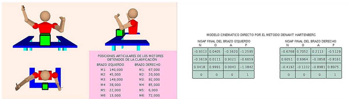
Figura 12: Resultado de la cinemática directa por parte del HMI. Fuente: Elaboración propia.
