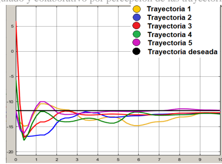
Figura 28: Perfil en Z de las 5 trayectorias del brazo izquierdo con control. Fuente: Elaboración propia.
