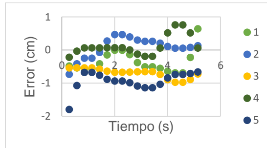
Figura 30: Error absoluto de los valores en X del brazo derecho con control. Fuente: Elaboración propia.
