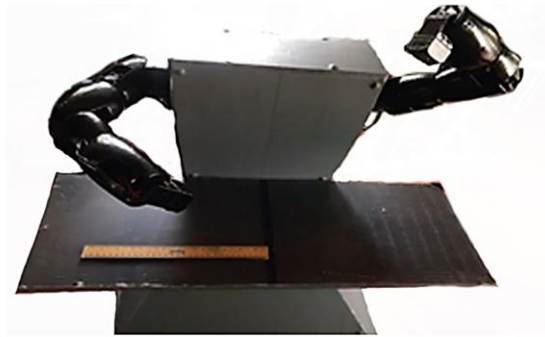
Figura 14: Posición de los manipuladores en una vista frontal para la validación del montaje físico. Fuente: Elaboración propia.
