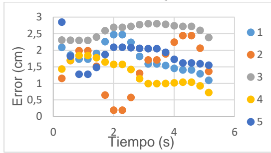
Figura 32: Error absoluto de los valores en Y del brazo derecho con control. Fuente: Elaboración propia.
