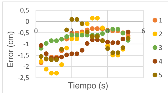
Figura 34: Error absoluto de los valores en Z del brazo derecho con control. Fuente: Elaboración propia.
