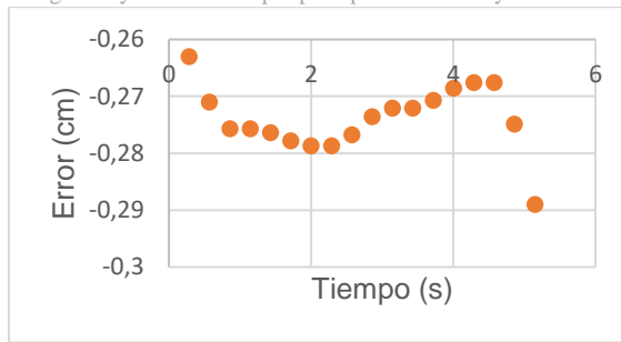
Figura 47: Error promedio de los valores de X del brazo izquierdo con control. Fuente: Elaboración propia.
