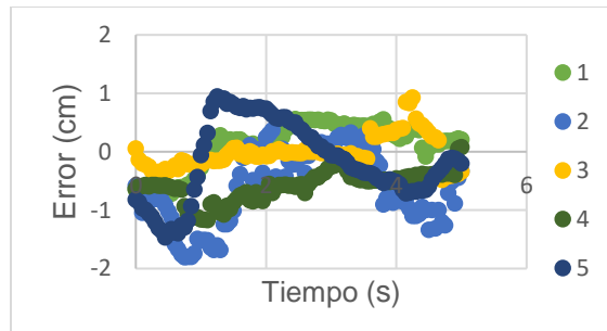
Figura 29: Error absoluto de los valores en X del brazo derecho. Fuente: Elaboración propia.
