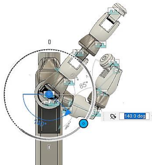
Figura 11: Diseño CAD de los manipuladores. Fuente: Elaboración propia.
