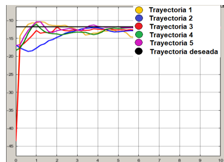
Figura 27: Perfil en Z de las 5 trayectorias del brazo izquierdo. Fuente: Elaboración propia.
