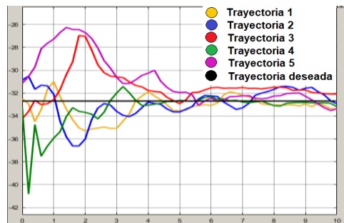
Figura 19: Perfil en Y de las 5 trayectorias el brazo derecho. Fuente: Elaboración propia.
