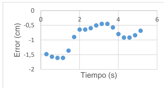
Figura 45: Error promedio de los valores en Z del brazo derecho con control. Fuente: Elaboración propia.
