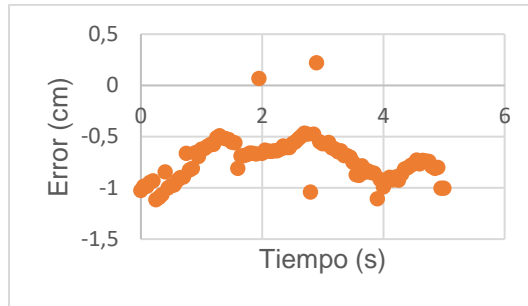
Figura 48: Error promedio de los valores de X del brazo izquierdo. Fuente: Elaboración propia.
