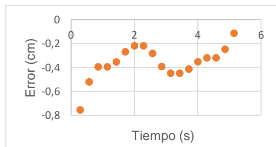
Figura 41: Error promedio de los valores de X del brazo derecho con control. Fuente: Elaboración propia.
