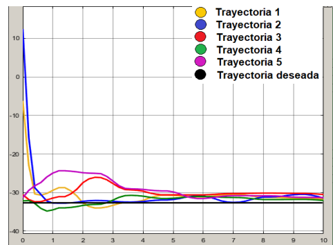
Figura 20: Perfil en Y de las 5 trayectorias del brazo derecho con control. Fuente: Elaboración propia.
