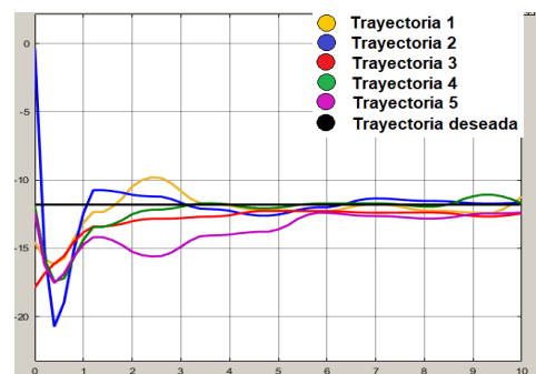
Figura 22: Perfil en Z de las 5 trayectorias del brazo derecho con control. Fuente: Elaboración propia
