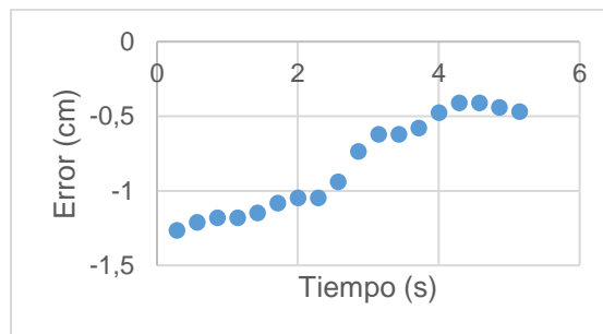
Figura 51: Error promedio de los valores en Z del brazo izquierdo con control. Fuente: Elaboración propia.
