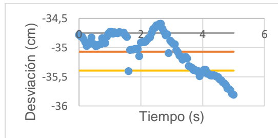
Figura 62: Desviación estándar de los valores en Y del brazo izquierdo. Fuente: Elaboración propia.
