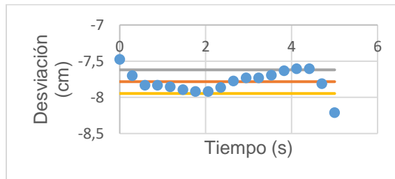
Figura 59: Desviación estándar de los valores en X del brazo izquierdo con control. Fuente: Elaboración propia.
