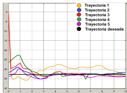
Figura 25: Perfil en Y de las 5 trayectorias del brazo izquierdo. Fuente: Elaboración propia.
