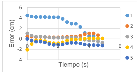
Figura 38: error absoluto de los valores en Y del brazo izquierdo con control. Fuente: Elaboración propia.
