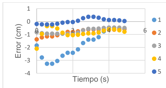
Figura 40: Error absoluto de los valores en Z del brazo izquierdo con control. Fuente: Elaboración propia.
