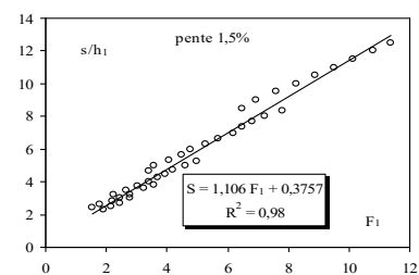
Figure 6 : Variation du rapport s/h_1 en fonction du nombre de Froude F_1 , pour \tan(\alpha) = 0,015 . (o) Points Expérimentaux
