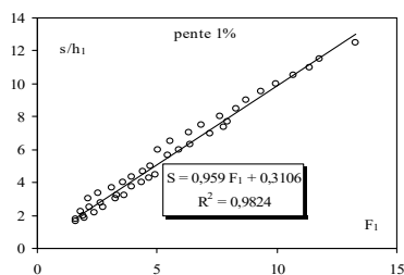
Figure 5: Variation du rapport s/h_1 en fonction du nombre de Froude F_1 , pour \tan(\alpha) = 0,01 . (o) Points expérimentaux
