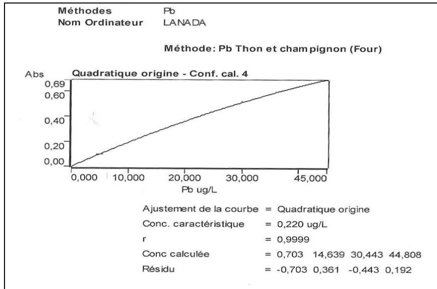
Figure 1: Courbe d'étalonnage du plomb.
