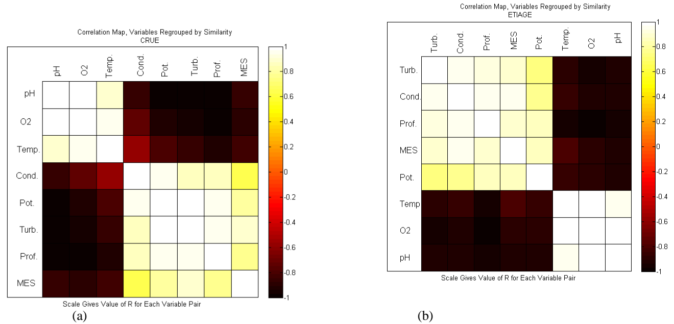
Figure 10: Matrice de corrélation des caractéristiques physicochimiques des eaux du lac d'Ayamé 1 ; a) : pendant la saison des pluies ; b) : pendant la saison sèche. Turb= Turbidité ; Temp= Température ; Cond= conductivité ; Pot= potentialité ; MES= Matières en suspension; Prof= Profondeur; O2=Oxygène dissous
