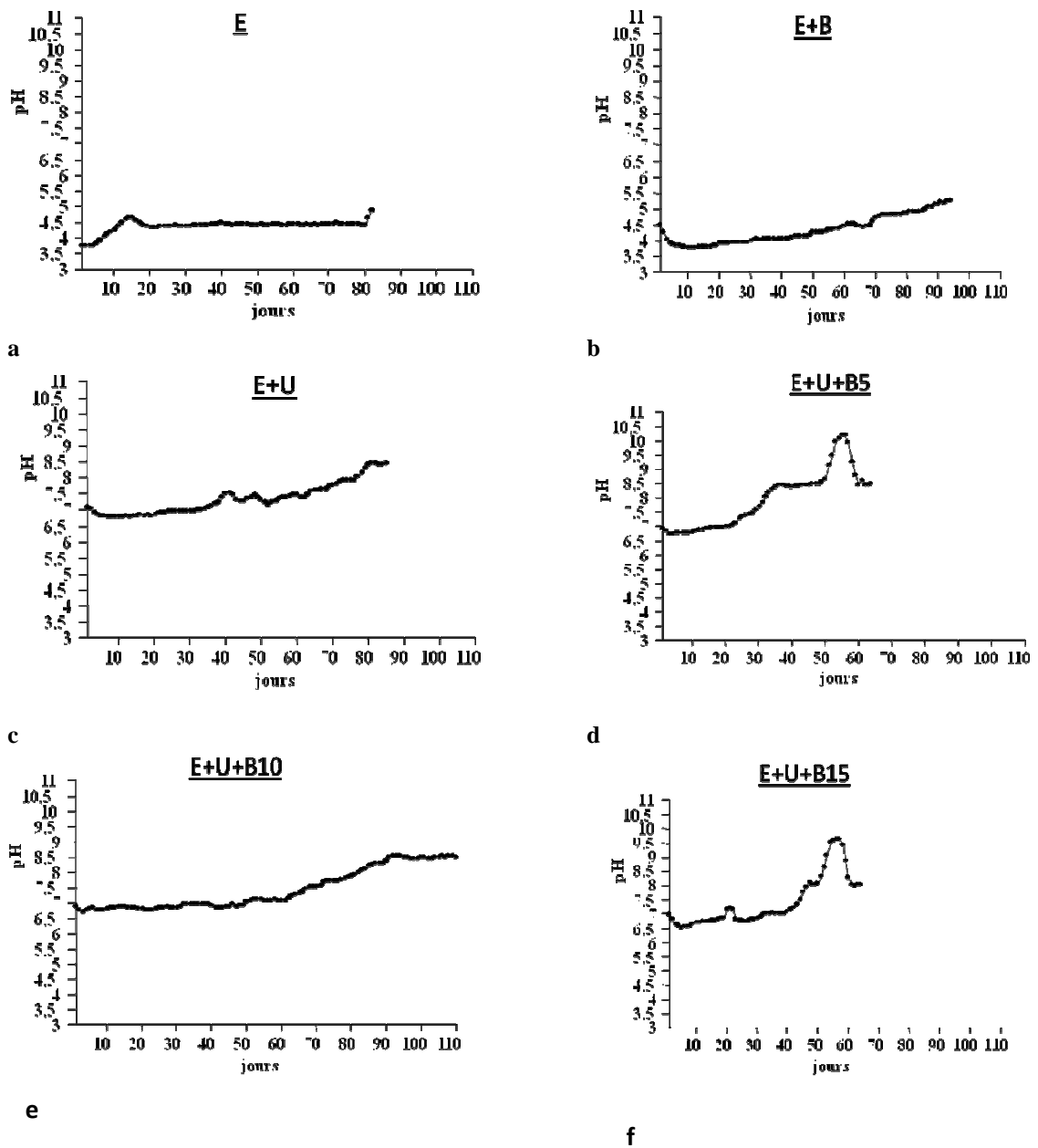
Figure 3 : Variation journalière du pH dans les différents réacteurs : a) réacteur 1, b) réacteur 2, c) réacteur 3, d) réacteur 4, e) réacteur 5, f) réacteur 6 ; E = effluent de manioc, E+B = effluents de manioc + 10 kg de bouse de vache, E+U = effluent de manioc + urine, E+U+B5 = effluents de manioc + urine + 5 kg de bouse de vache, E+U+B10 = effluents de manioc + urine + 10 kg de bouse de vache, E+U+B15 = effluents de manioc + urine + 15 kg de bouse de vache.
