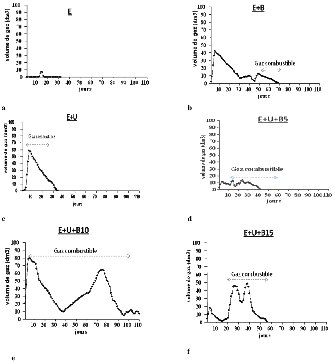
Figure 4 : Variation journalière de la production de gaz par les différents réacteurs : a) réacteur 1, b) réacteur 2, c) réacteur 3, d) réacteur 4, e) réacteur 5, f) réacteur 6 ; E = effluent de manioc, E+B = effluents de manioc + 10 kg de bouse de vache, E+U = effluent de manioc + urine, E+U+B5 = effluents de manioc + urine + 5 kg de bouse de vache, E+U+B10 = effluents de manioc + urine + 10 kg de bouse de vache, E+U+B15 = effluents de manioc + urine + 15 kg de bouse de vache.
