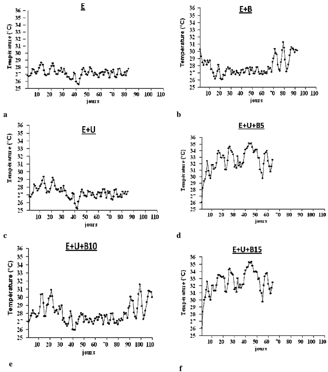
Figure 2 : Variation journalière de la température dans les différents réacteurs : a) réacteur 1, b) réacteur 2, c) réacteur 3, d) réacteur 4, e) réacteur 5, f) réacteur 6 ; E = effluent de manioc, E+B = effluents de manioc + 10 kg de bouse de vache, E+U = effluent de manioc + urine, E+U+B5 = effluents de manioc + urine + 5 kg de bouse de vache, E+U+B10 = effluents de manioc + urine + 10 kg de bouse de vache, E+U+B15 = effluents de manioc + urine + 15 kg de bouse de vache.
