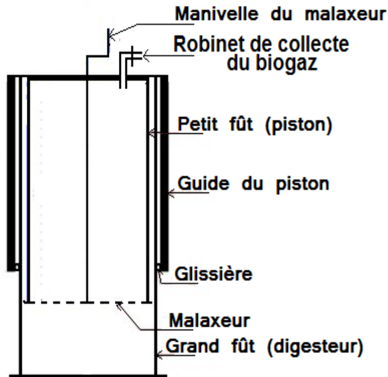
Figure 1 : Schéma présentant une vue de profil du digesteur expérimental.
