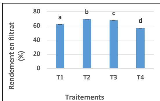
Figure 3: Rendement en filtrat du filtre-presse
