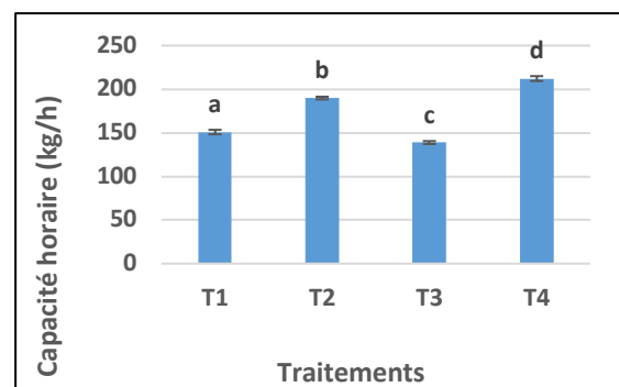
Figure 4: Capacité horaire du filtre-presse
