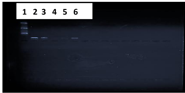
Lane 1 – DNA ladder; Lane 2 – N. meningitidis (DNA purity @ A_{260}/A_{280} - 1.53); Lane 3 – H. influenzae (DNA purity @ A_{260}/A_{280} - 1.48); Lane 4 – S. pneumoniae (DNA purity @ A_{260}/A_{280} - 1.57); Lane 5 - N. meningitidis (DNA purity @ A_{260}/A_{280} - 1.53); Lane 6 - H. influenzae (DNA purity @ A_{260}/A_{280} - 1.48)
