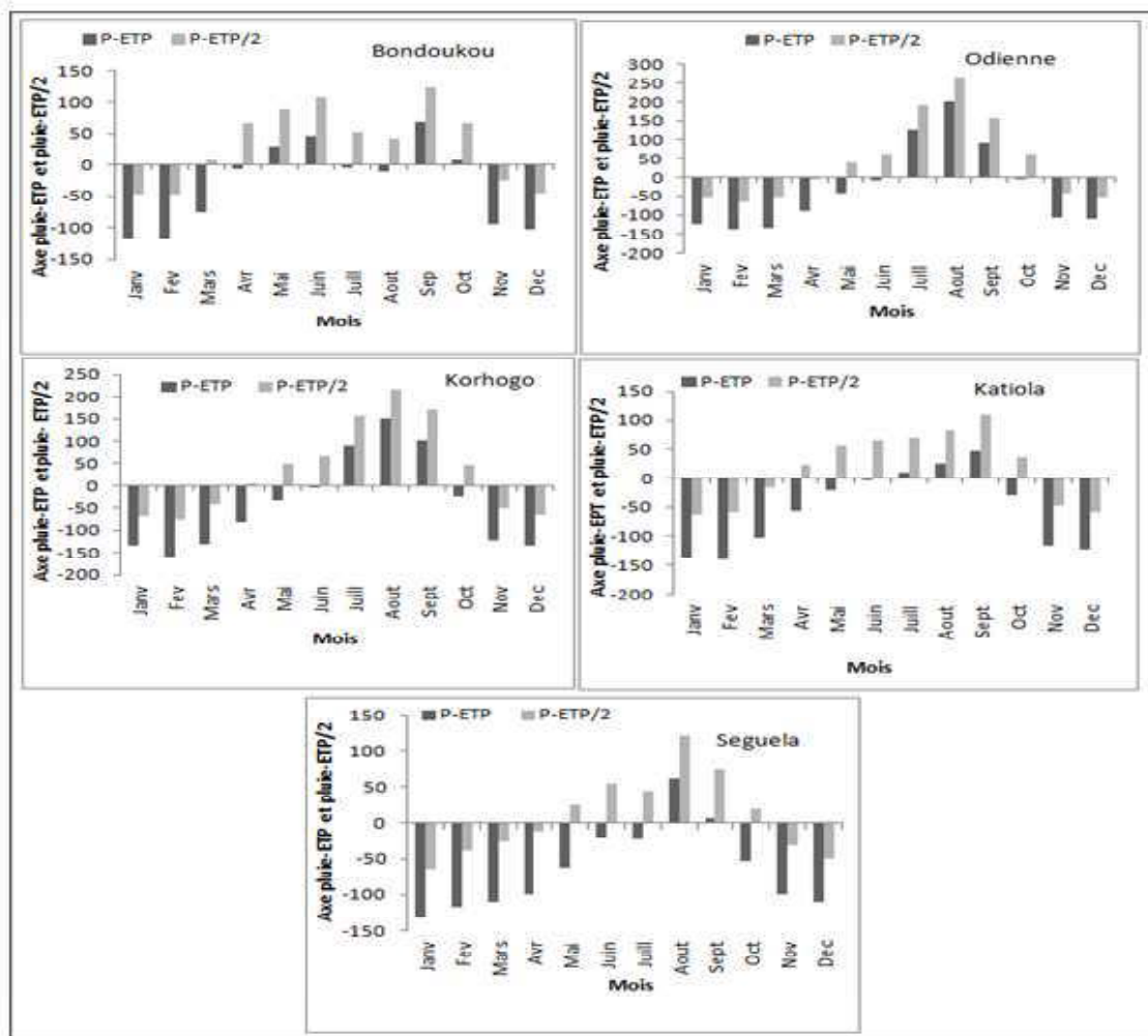
Figure 3 : Bilan climatique par localité de la zone étudiée, après les dates de rupture.
