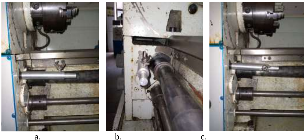
Gambar 3. Pemasangan ESL Pada Mesin Bubut Tipe Basic Plus 100809 a. Tampak Samping b. Tampak Depan c. Tampak Atas
