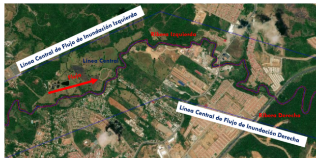
Esquemático del área del estudio realizado Fuente: Ing. Ricardo De León.
