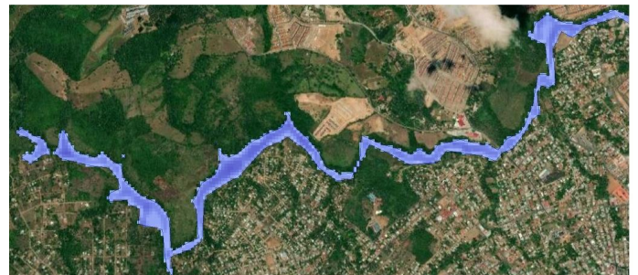
Planicie de Inundación Generada presentando las profundidades de agua por encima del terreno inundado
