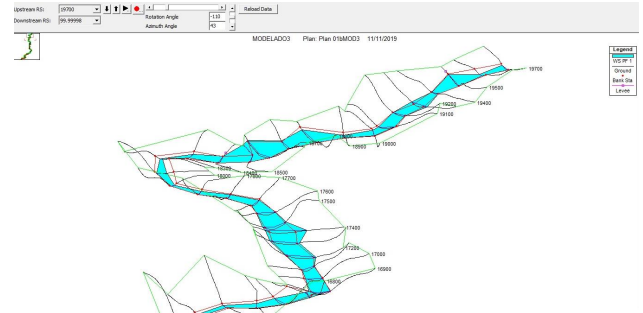
Resultados del Hec-Ras Fuente: Ing. Ricardo De León
