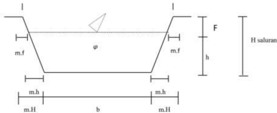
Gambar. 1 Dimensi penampang untuk saluran sekunder.
