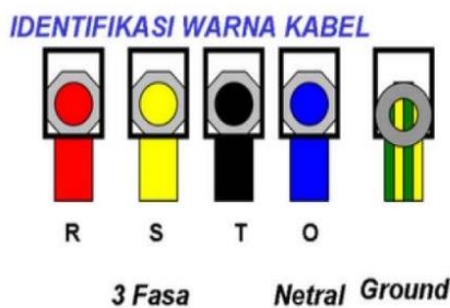
Gambar 1. Rangkaian Fasa
