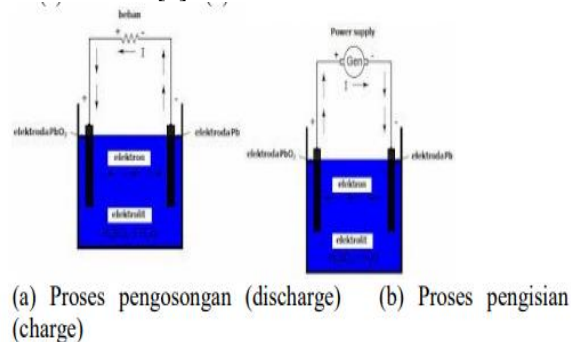
Gambar 13. Arah aliran elektron dan arus listrik pada baterai
