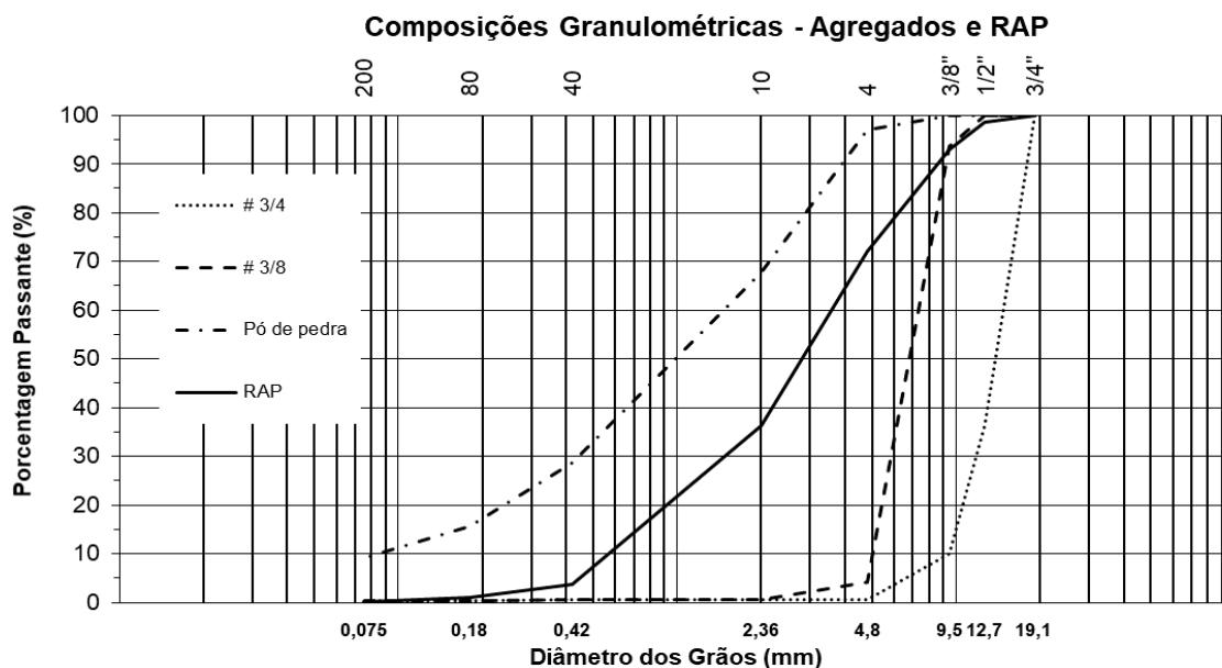
Figura 2. Granulometrias encontradas dos materiais agregados e RAP
