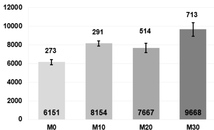
Figura 7. Resultados médios e desvios padrão de Módulo de Resiliência
