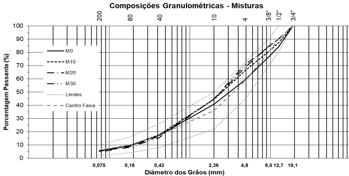
Figura 3. Curvas granulométricas das misturas asfálticas
