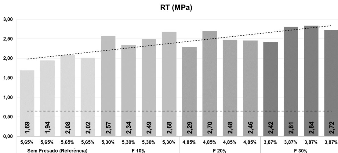
Figura 4. Resultados de resistência a tração
