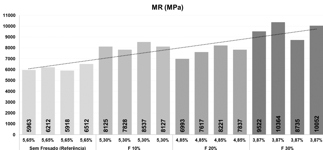
Figura 6. Resultados de módulo de resiliência
