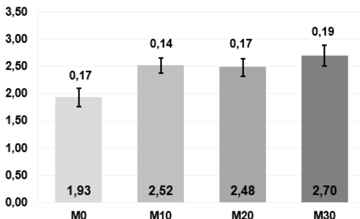
Figura 5. Resultados médios e desvios padrão de resistência a tração
