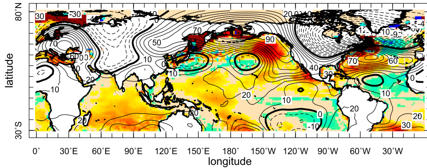
NCEP-NCAR NDJFMA 2013-2014
