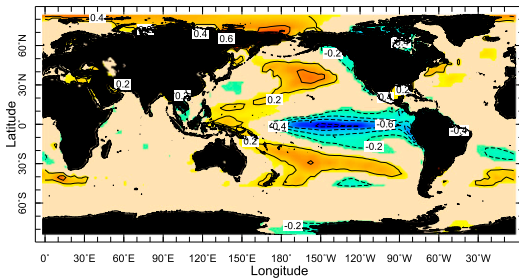
ESRL-GFSv2
