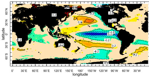
CCM3
