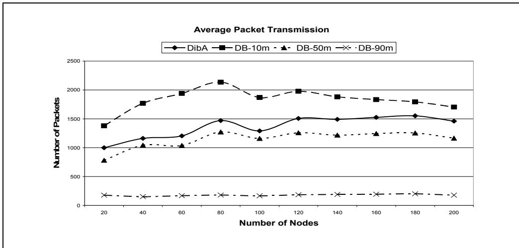
Fig. 22. APT - Diverse - BGR 60p/s
