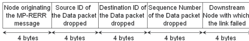
Fig. 26. Multi-path Route Error (MP-RERR) Message
