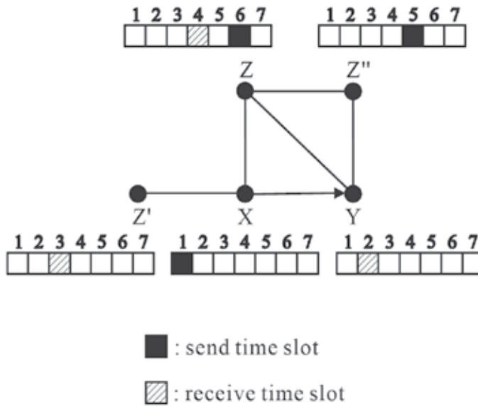
Fig. 4. An example of Lemma 1.
