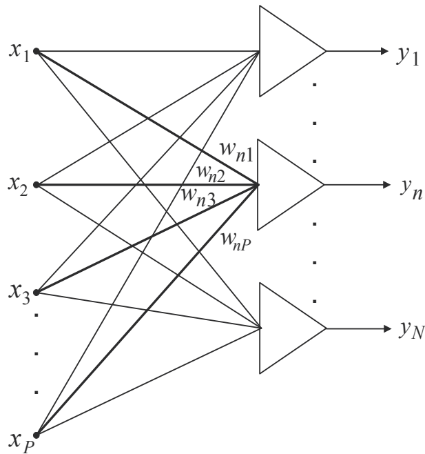
Fig. 7. SOM neural network
