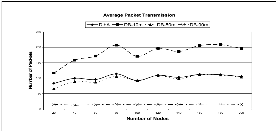
Fig. 16. APT - Diverse - BGR 5p/s
