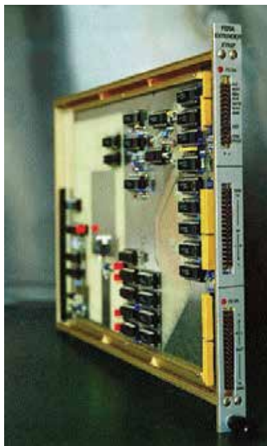
Fig. 2. FERA Extender/Tagger module.
