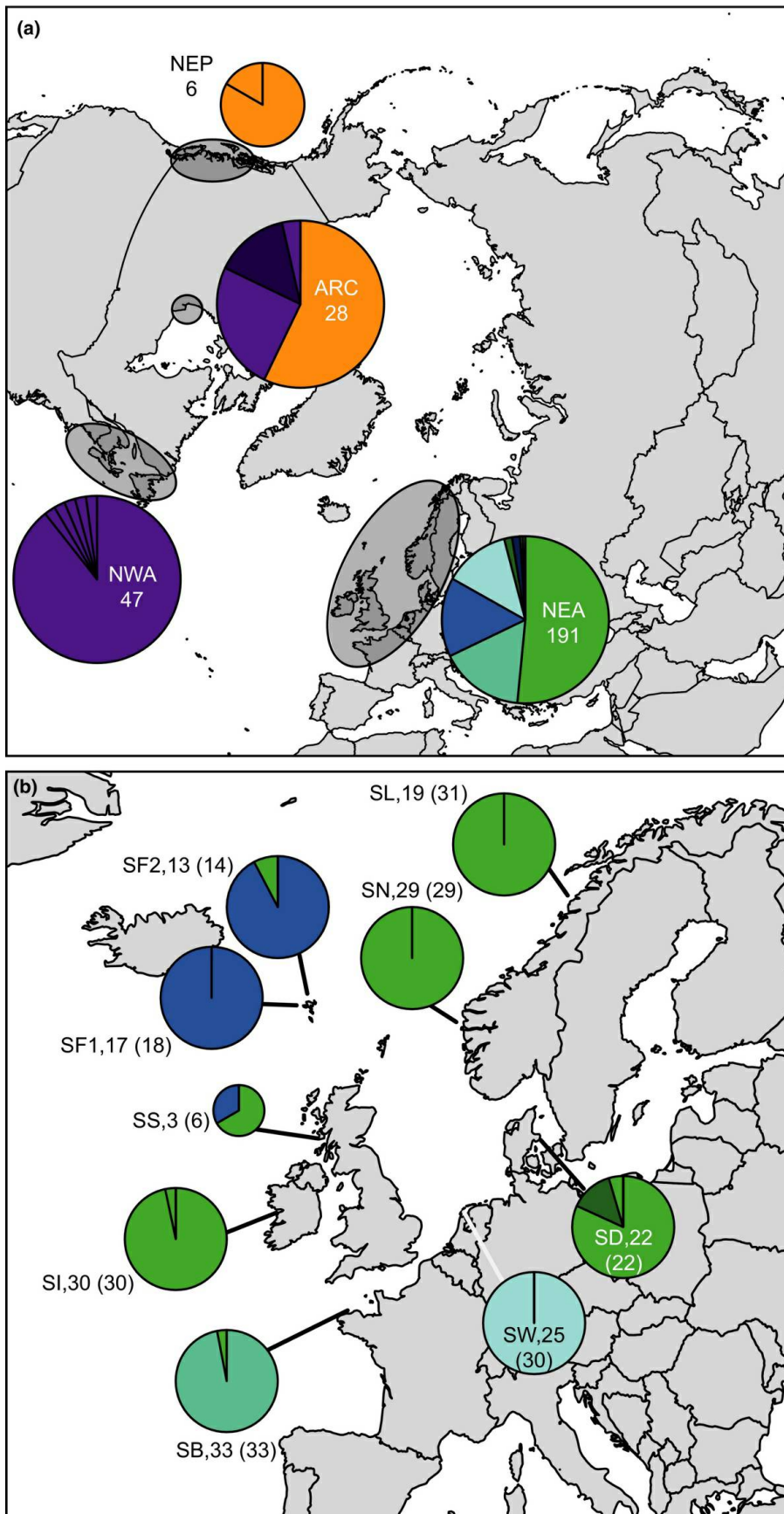
Figur 12. Innsamlingssteder og resultater ved bruk av mitokondrielt DNA (cytochrome-c-oxidase I) av sukkertare. Forkortelser er de samme som i figur 3, i tillegg SF2 som er dyrket materiale fra Færøylene (Figuren er fra Luttikhuisen et al. (2018)).
