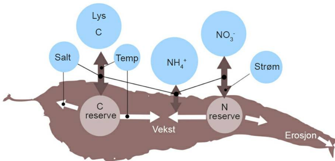
Figur 1. Skematisk oversikt over de viktigste faktorene som trengs for vekst hos makroalger med sukkertare som eksempel. Modifisert etter Broch et al. 2019. Reserve C og N blir næring for andre og kan høstes.
