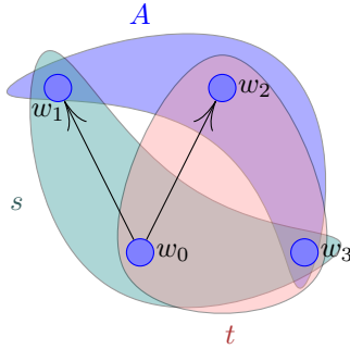
Figure 2.: Example for s : A \wedge t : A \wedge s \hat{+} t : A \wedge s \hat{-} t : A \wedge s \cup t : A \not\vdash s + t : A .
