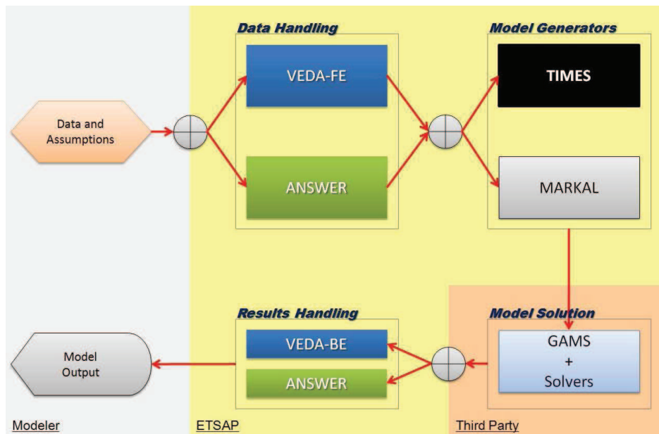
Figure 4.4 : Principe de fonctionnement de la modélisation VEDA-TIMES
