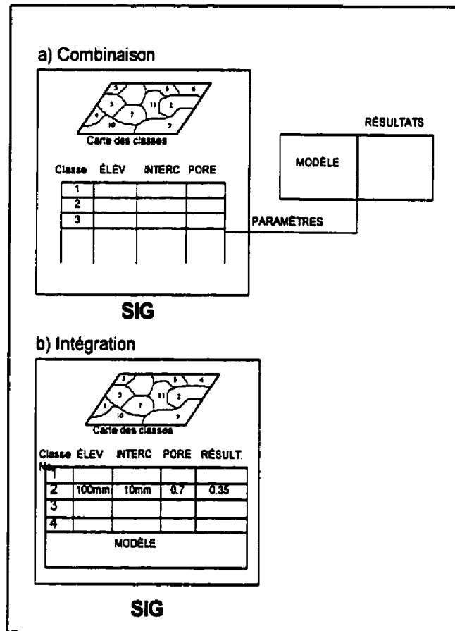
Figure 2.3 Deux idéologies en matière de lien entre un système d'information géographique et un modèle hydrologique (Stuart et Stocks, 1993)
