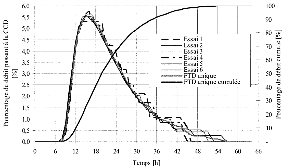
Figure 6.3 : Résultats des six essais et de la FTD unique
