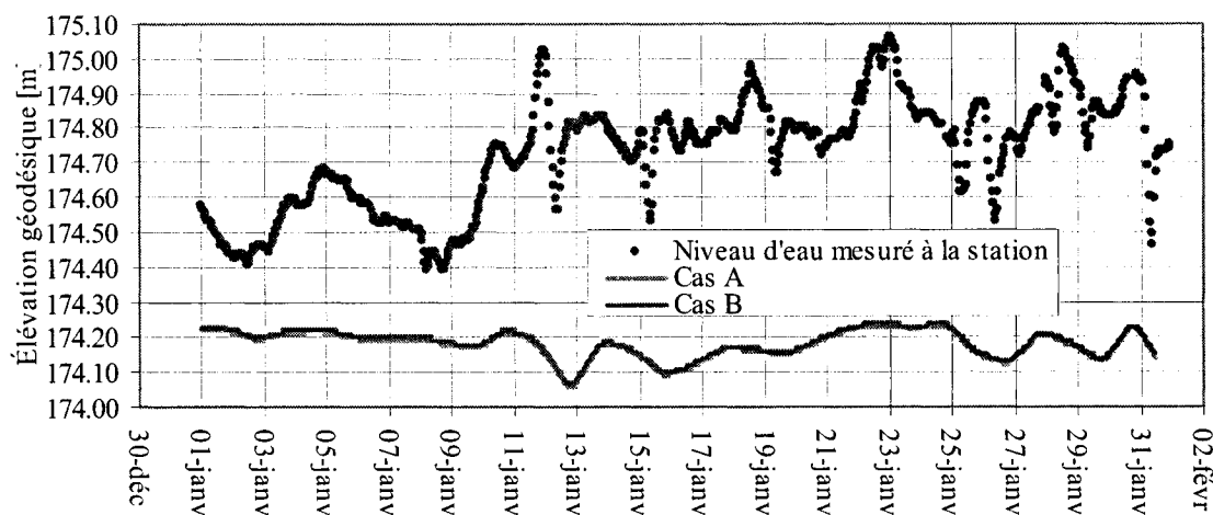
Figure 5.8 : Simulation en période hivernale – janvier 2003 – PK 150,6
