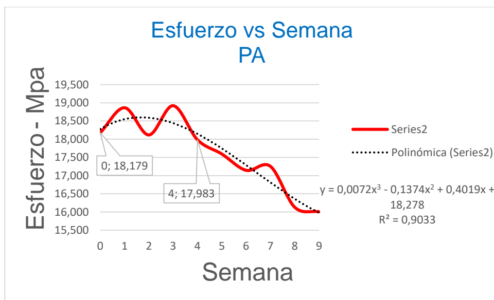
Figura 24 Diagrama esfuerzo-semana probetas de alcohol
