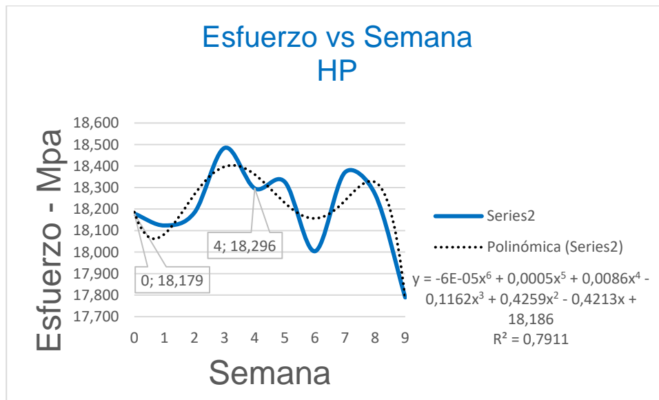
Figura 26 Diagrama esfuerzo-semana probetas de hipoclorito
