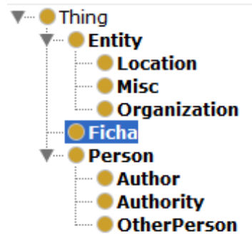
Figura 4. Jerarquía de clases de la ontología.
