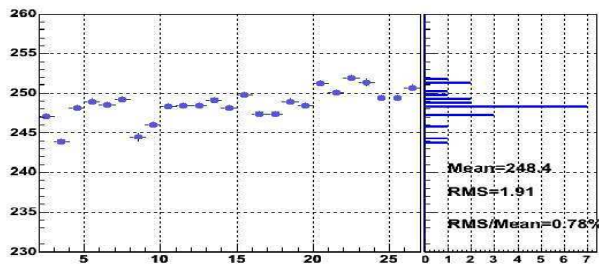
FIG. 20.8 – Réponse en énergie en fonction du numéro des cellules du compartiment milieu
