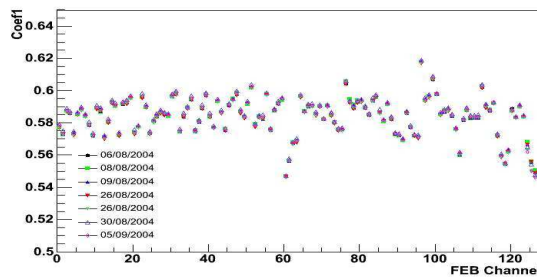
FIG. 20.6 – Coefficient de calibration r1 pour une FEB dans le compartiment milieu pour différentes prises de données.
