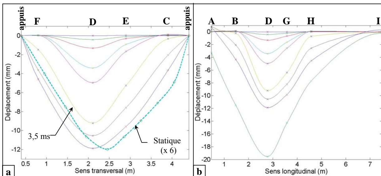
figure III.29 : évolution de la déformée (a) dans le sens transversal et (b) dans le sens longitudinal pour des pas de temps après contact de 0,57 ms ; 1 ms ; 1,5 ms ; 2 ms ; 3,5 ms ; 5 ms ; 6,7 ms et 15,3 ms (uniquement pour la figure b - déplacement maximal) – Test T4
