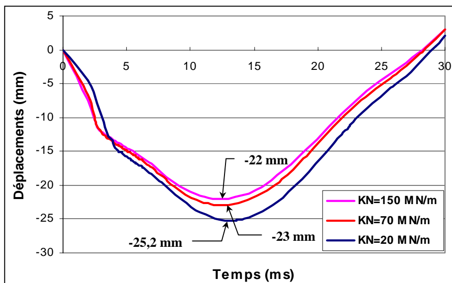
figure V.13 : variation du déplacement au point d'impact en fonction du paramètre de contact « KN »
