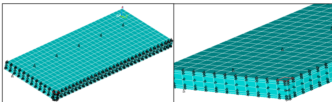
figure V.8 : modèle statique sous ANSYS
