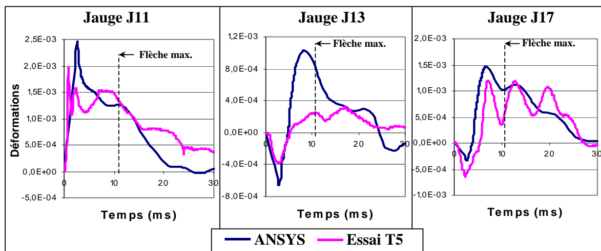
figure V.16 : comparaison des déformations expérimentales et sous ANSYS des armatures inférieures pour l'essai T5– J11 à 0,34 m du point d'impact, J13 à 1,15 m et J17 à 1,34 m
