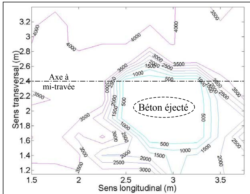
figure III.35 : résultats de l'analyse par ultrasons après le test T6 (vitesse en m.s^{-1} )
