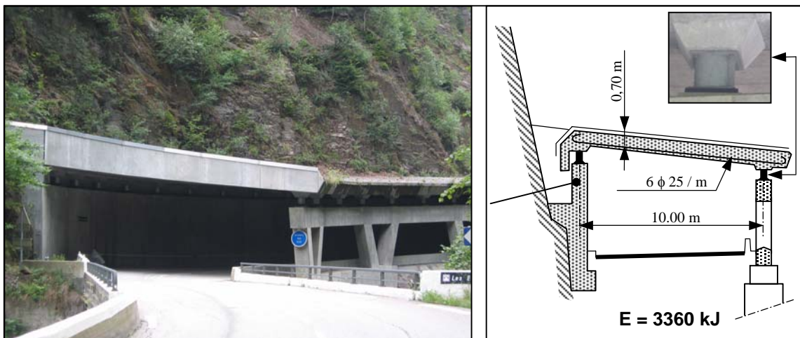
figure I.7 : Pare-blocs Structurellement Dissipant des Essariaux (Val d'Arly - Savoie)
