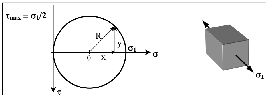
figure IV.23 : cercle de Mohr dans le cas d'un chargement uniaxial en traction
