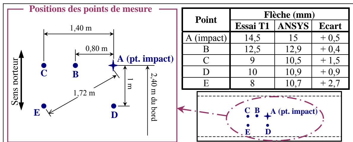
figure V.19 : déplacements verticaux en sous face de dalle pour l'essai T1
