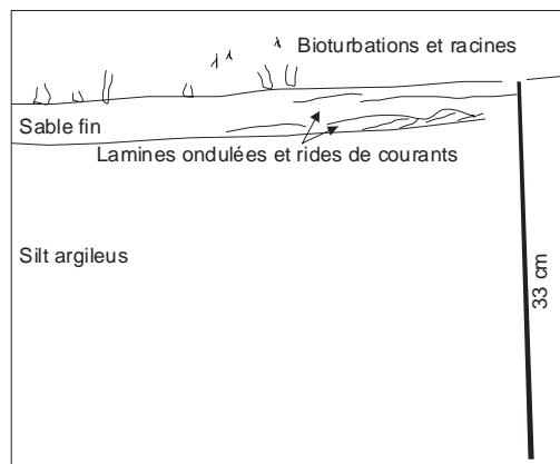
Figure 2.19 : faciès de Thimi. A) Faciès 2: sable et silt : faciès de comblement en environnement de front de delta, B) Faciès 3: comblement en environnement de plaine deltaïque par une rivière en méandres et C) Faciès 9: comblement et environnement tidal.
