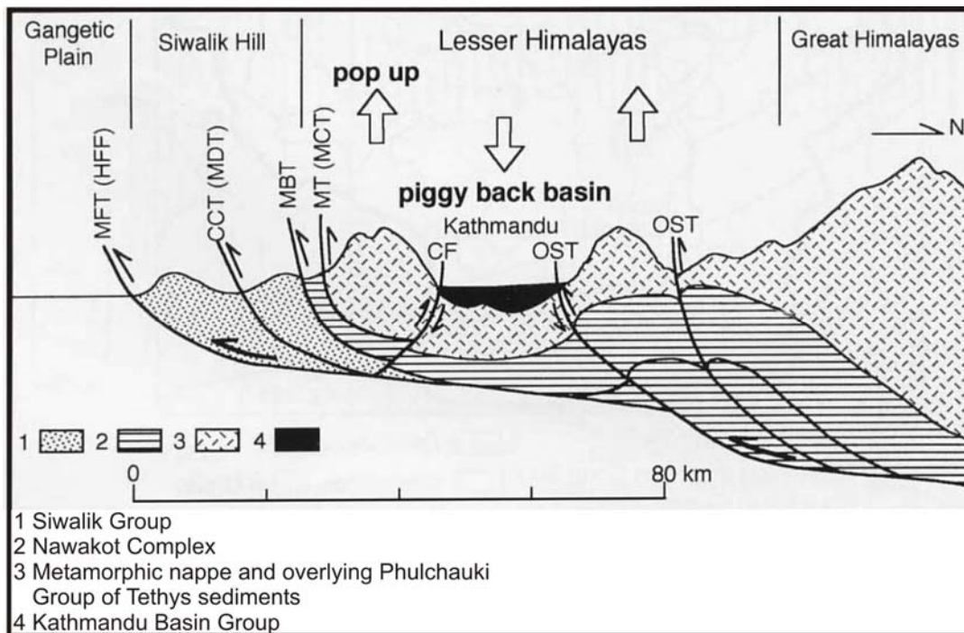
Figure 3.18: coupe de la structure crustale sous le bassin de Kathmandu, suggérant que le MBT se raccorde au décollement basal sous la partie sud du bassin de Kathmandu et que la faille de Chandragiri recoupe tardivement les structures. (OST: chevauchement hors séquence à l'avant du front morphologique du Haut Himalaya; CF Faille de Chandragiri (D'après Sakai, 2001a), p.6.
