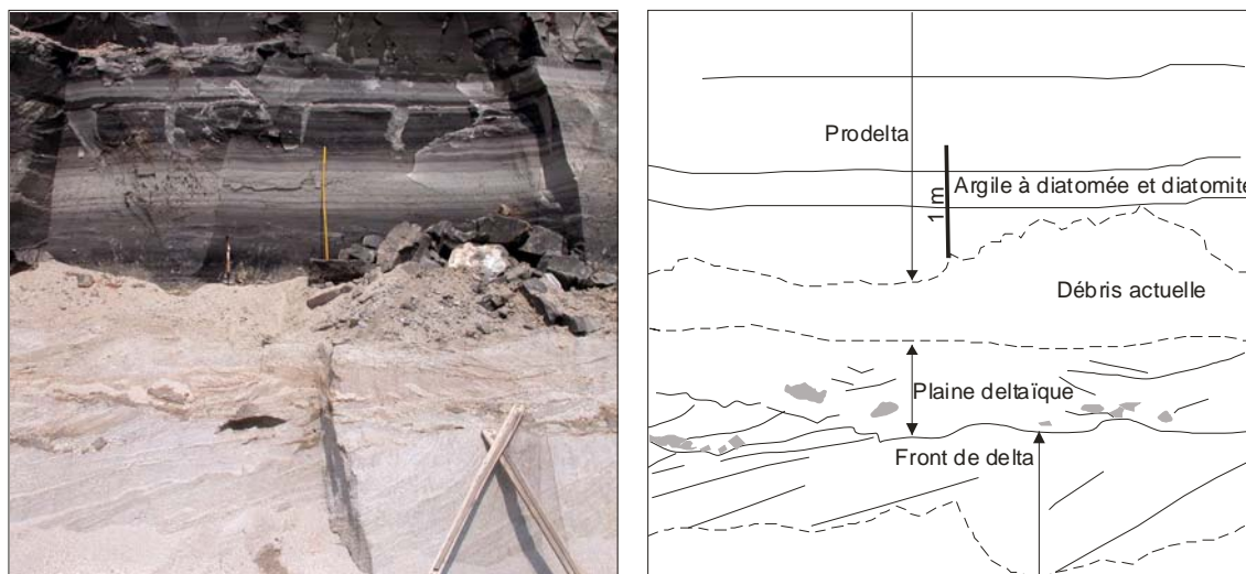
Figure 2.9 : affleurement d'argiles à diatomées et diatomites, faciès de prodelta (base de la formation Lgd, coupe Balaju 2, voir Fig. 2.12).
