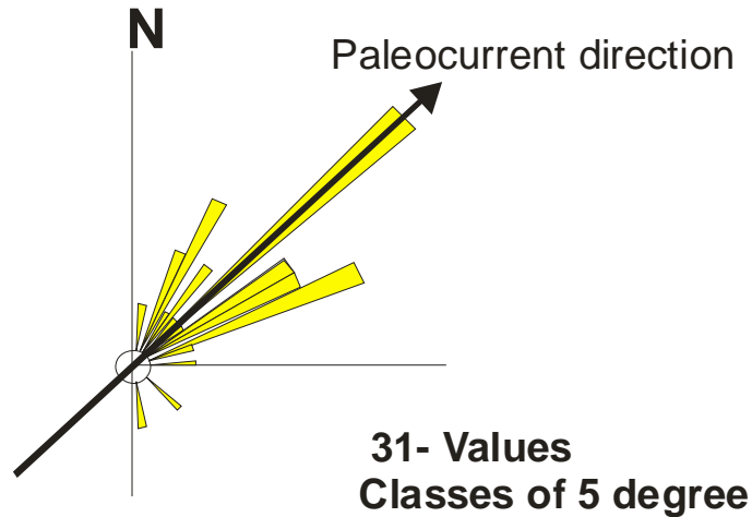
Figure 3.4 : analyse des directions des paléo-courants à Koteswor (directions déduites des laminations).
