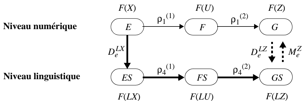
Fig. 40 : Chaînage de règles.
