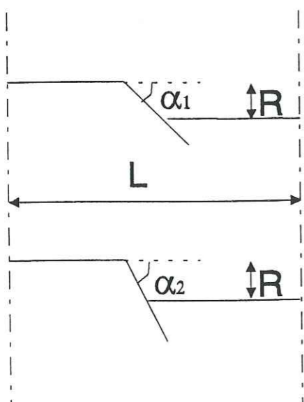
Figure 105: Si on veut allonger la longueur de socle ( L_s ) sans changer la longueur de la coupe ( L ), il faut augmenter le pendage des failles.
