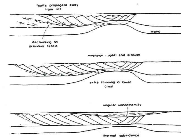
Modèle de Coward (1986)
