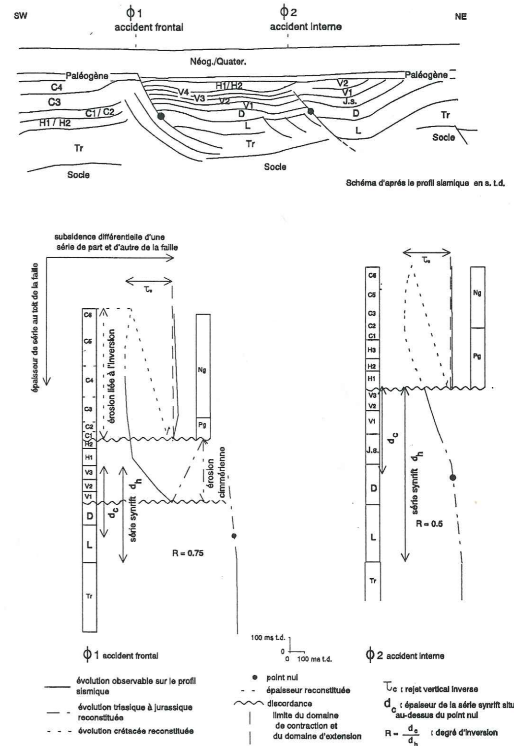
Figure 65 : Diagramme d'analyse de subsidence différentielle le long d'une coupe transverse à la bordure SW (voir localisation fig. 69).
