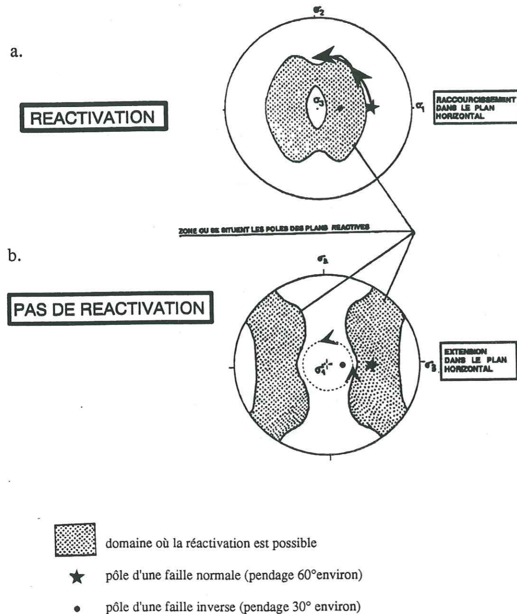
Figure 23 : Effet de l'obliquité entre l'azimut de la faille et le trièdre des contraintes pour R = 0,55 ; \phi_f = 34^\circ et \sigma_3 = 0,1\sigma_1 .
