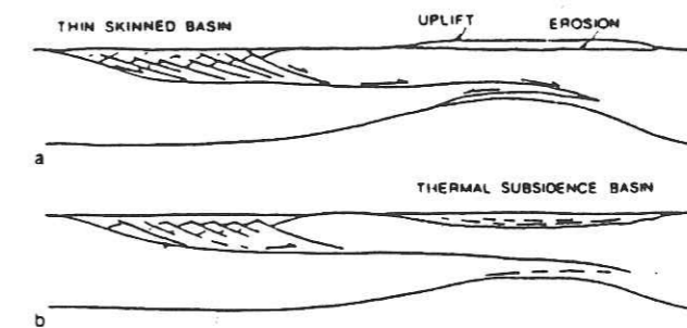
Modèle de Wernicke (1985)
