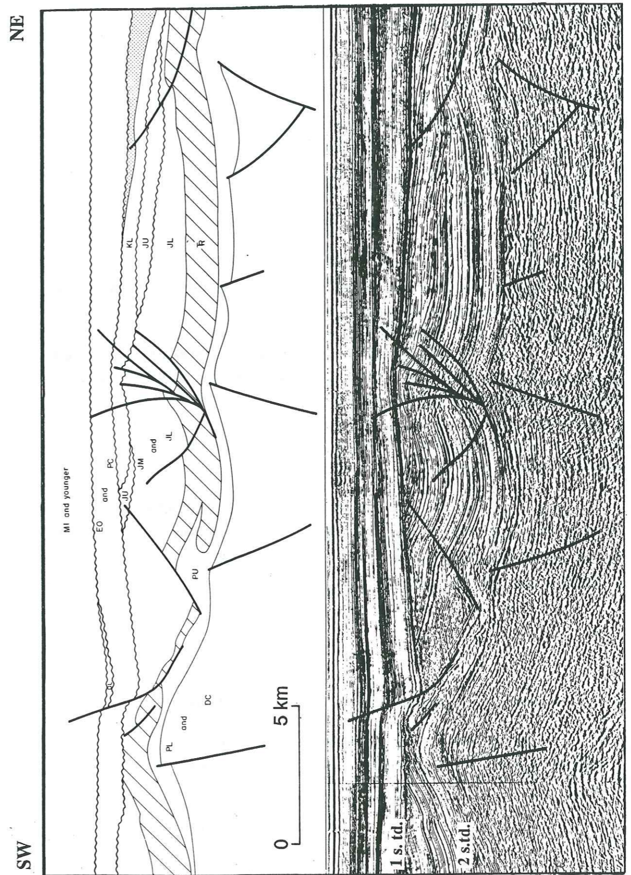
Figure 40 : Profil sismique (le Nord du Broad Fourteens Basin) illustrant la discordance cimmérien moyen et la discordance cimmérien tardif. Notez l'épaissement important du Jurassique au SW du profil (d'après van Wijhe, 1987).
