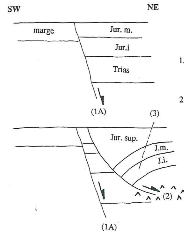
Figure 107 : schéma d'une évolution possible des failles (1A), (2), et (3)
