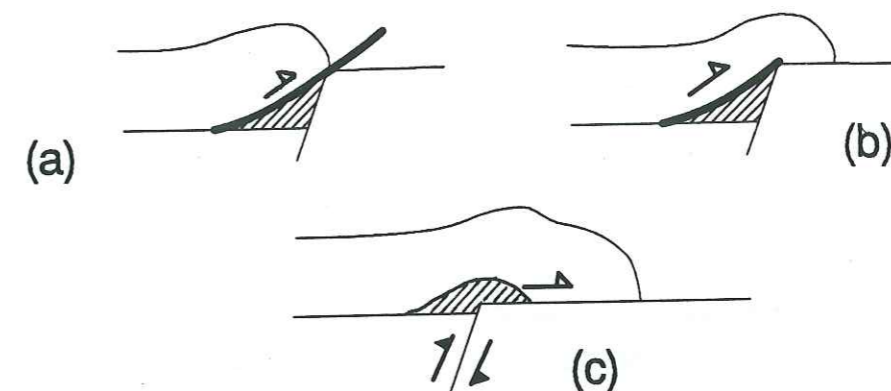
Figure 90 : Formation d'une écaille en pied de faille normale
