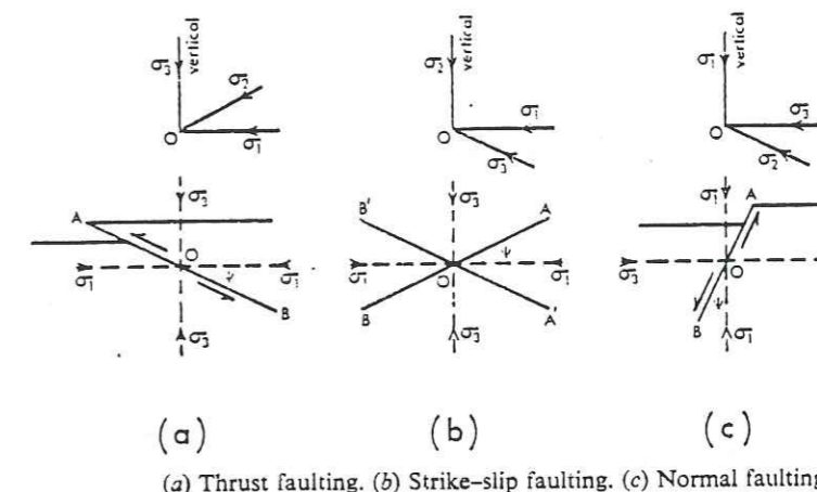
Figure 13a : Classification des types de failles selon Anderson (d'après Jaeger et Cook, 1969). (a) et (c) sont des coupes alors que (b) correspond à une vue en plan.
