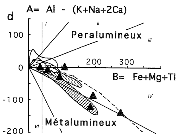
FIG. 44 - Distribution des orthogneiss de Bolocho dans les diagrammes K 2 O vs SiO 2 (a), QP (b), QBF (c), AB (d) et Mg*B (e). Explications dans le texte et fig. 33.
