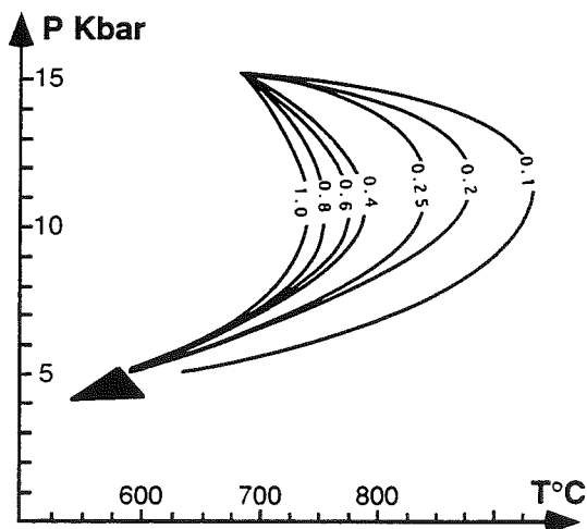
FIG. 21 - Calcul de chemins rétrogrades théoriques en fonction du taux de dénudation pour des éclogites du Massif Central. D'après Mercier et al. [1991]. Paramètres utilisés:
