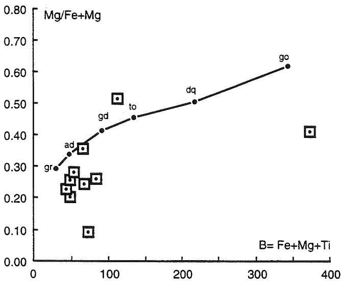
FIG. 56 - Distribution des échantillons d'Hemasil dans le diagramme Mg/Fe+Mg vs B de Debon et Le Fort [1988]. Paramètres calculés en millications pour 100 g de roche. Compositions moyennes de référence, cf. fig. 55 pour les abréviations. La ligne passant par les points de référence est utilisée pour distinguer les associations magnésiennes, communes et ferrifères. A l'exception de TK837, les roches d'Hemasil présentent un caractère plutôt ferrifère.
