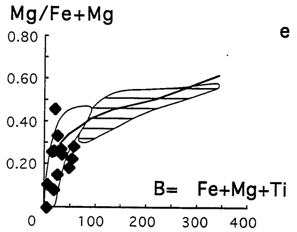
FIG. 34 - Distribution des orthogneiss de la Basha dans les diagrammes K 2 O vs SiO 2 (a), QP (b), QBF (c), AB (d) et Mg*B (e). Explications dans le texte et fig. 33.
