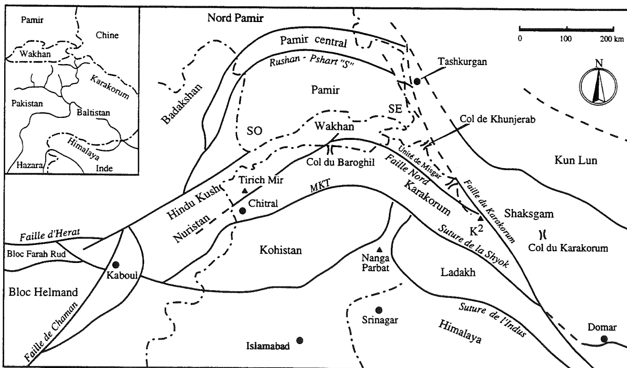
FIG. 7 - Les principales sutures dans le Karakorum et le Pamir. D'après Le Fort et al. [1994].
