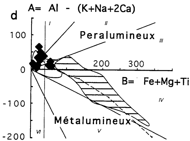
FIG. 34 - Distribution des orthogneiss de la Basha dans les diagrammes K 2 O vs SiO 2 (a), QP (b), QBF (c), AB (d) et Mg*B (e). Explications dans le texte et fig. 33.
