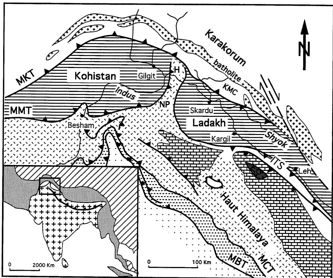
FIG. 2 - Carte géologique simplifiée de la partie Nord-Ouest de l'orogène himalayen.
