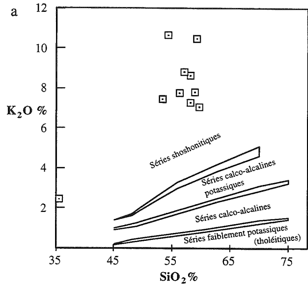
FIG. 55 - Diagramme K_2O vs SiO_2 (a) et K_2O vs Na_2O (b) des échantillons de syénite et de TK838. L'amphibolite TK489 n'est pas représentée. Ces roches correspondent à une association shoshonitique évoluant vers des termes ultra-potassiques.
