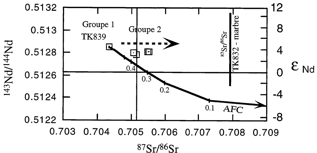
FIG. 64 - Diagramme ^{143}\text{Nd}/^{144}\text{Nd} vs ^{87}\text{Sr}/^{86}\text{Sr} de la syénite d'Hemasil et essai de modélisation de processus d'AFC [DePaolo, 1981]. Le contaminant choisi correspond à la composition moyenne de la croûte supérieure de Zartman et Haines [1988]. Les chiffres reportés sur la courbe d'AFC correspondent à la fraction de liquide restant (paramètre F). Pour l'AFC, les paramètres utilisés sont: vitesse d'assimilation/vitesse de cristallisation r = 0,2 ; coefficients de partage minéral/liquide D_{\text{Nd}} = 2 et D_{\text{Sr}} = 1,5 . Le rapport ^{87}\text{Sr}/^{86}\text{Sr} du carbonate encaissant (échantillon TK832) a également été reporté. Une assimilation de Sr radiogénique en provenance de cet encaissant lors de la mise en place du pluton peut expliquer la dispersion observée.
