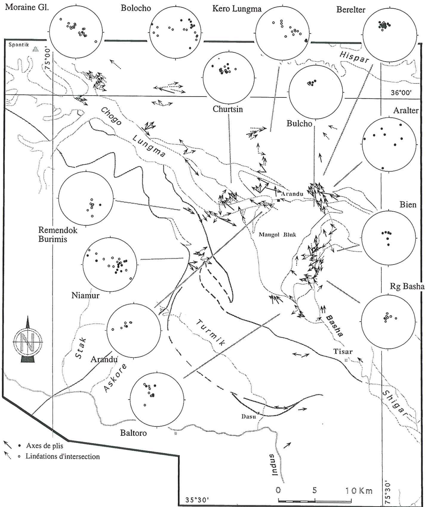
FIG. 10 - Carte des linéations d'intersections et des axes plis et projections stéréographiques par secteur (Wulff, hémisphère inférieure).
