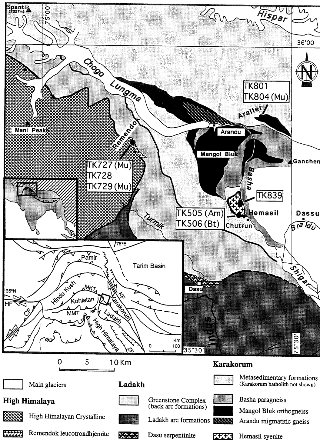
FIG. 66 - Carte géologique simplifiée du secteur du Chogo Lungma et localisation des échantillons. KF: Karakorum Fault; MKT: Main Karakorum Thrust; MMT: Main Mantle Thrust; ZF: Zanskar Fault; HF: Herat Fault; CF: Chaman Fault.
