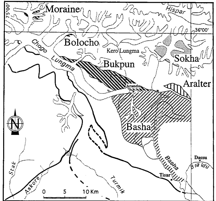
FIG. 26 - Carte de localisation des différents groupes d'orthogneiss.
