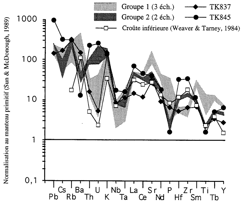
FIG. 58 - Diagramme multi-éléments normalisé au manteau primitif [Sun et McDonough, 1989] des échantillons de syénite et du lamprophyre. Cf. texte pour la distinction des différents groupes. Une composition moyenne de croûte inférieure [Weaver et Tarney, 1984], a été ajoutée pour comparaison. Cette dernière est particulièrement enrichie en Ba par rapport au manteau primitif et présente une anomalie négative en U-Th prononcée.
