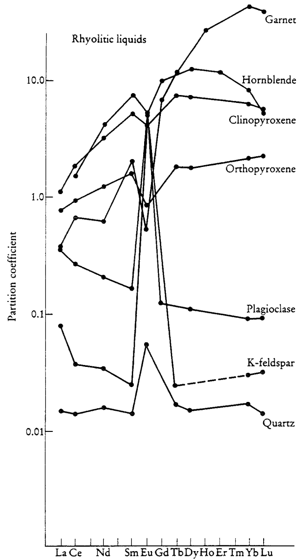
FIG. 37 - Coefficients de partage minéral/liquide des terres rares dans les minéraux communs des magmas rhyolitiques. D'après Rollinson [1993].
