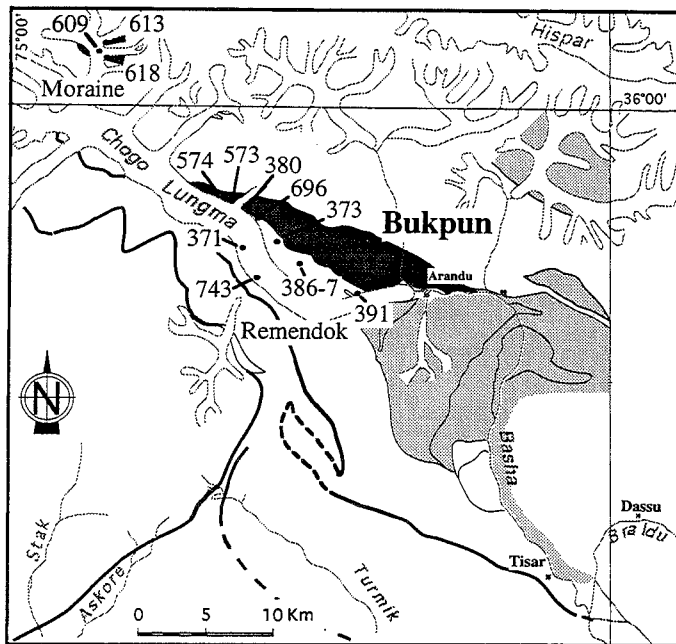
FIG. 28 - Carte de localisation des orthogneiss du Bukpun.
