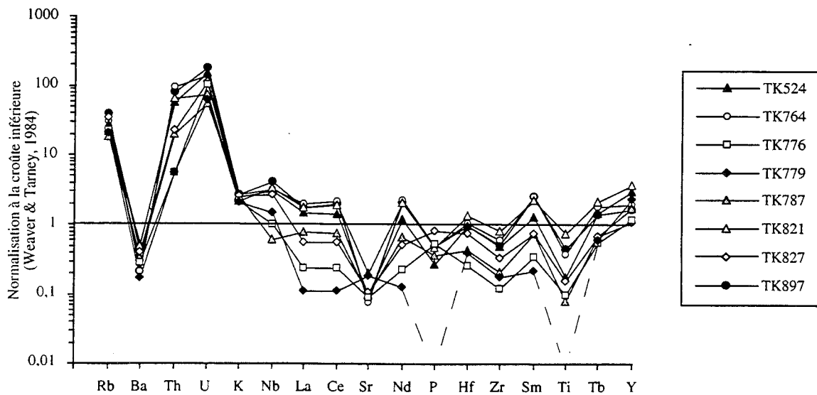
FIG. 38 - Diagramme multi-éléments normalisé à la croûte inférieure des orthogneiss de la Basha.
