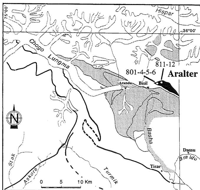
FIG. 29 - Carte de localisation des orthogneiss d'Aralter.
