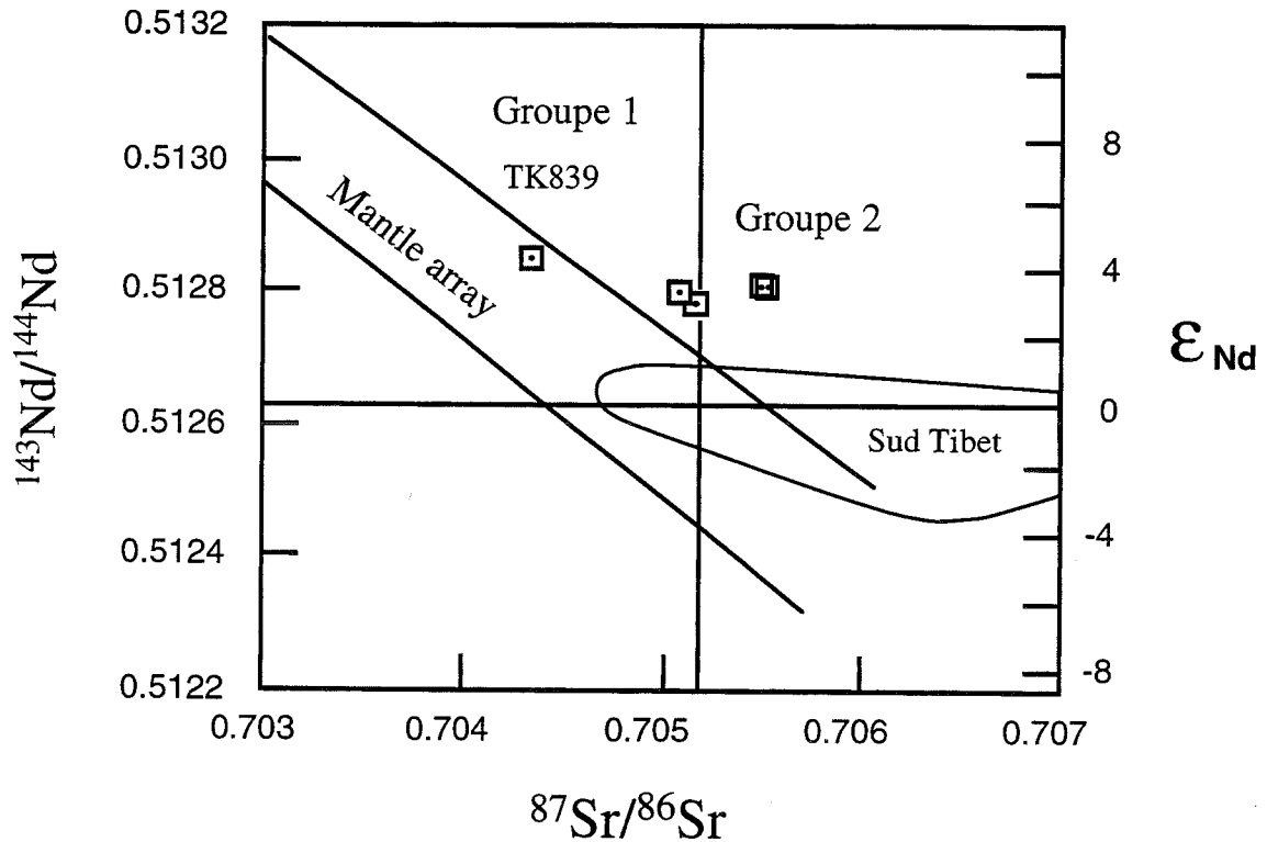
FIG. 63 - Diagramme ^{143}\text{Nd}/^{144}\text{Nd} vs ^{87}\text{Sr}/^{86}\text{Sr} des échantillons de syénite. Les champs correspondant aux volcanismes shoshonitiques du plateau du Tibet ont été reportés [Turner et al. , 1996].
