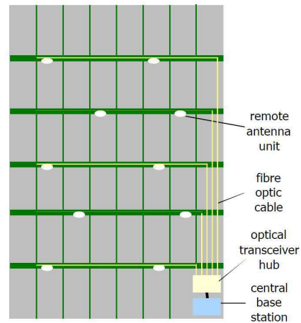
FIGURE 1.1 – Schéma représentatif du principe de RoF en intérieur (issu de [14]).
