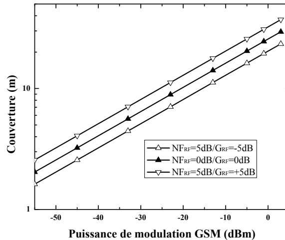
FIGURE 3.14 – Résultats en couverture GSM en fonction de la puissance de modulation du VCSEL, pour un exposant de pertes de propagation n valant 5 et pour différents front-ends RF.
