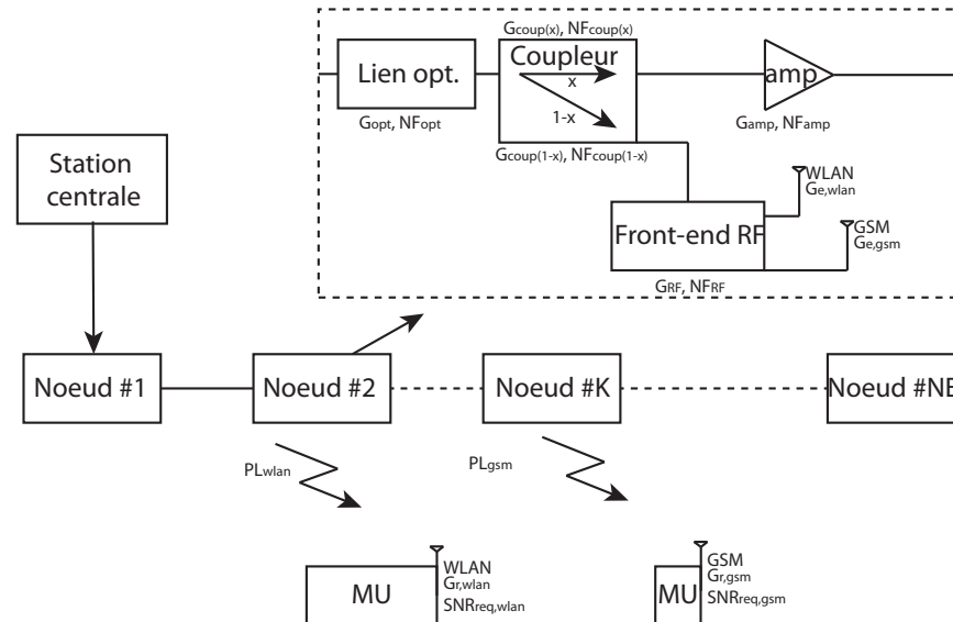
FIGURE 3.22 – Proposition de système associé à notre tunnel optique pour une utilisation dans une architecture de type bus dans le cadre d'une liaison descendante.
