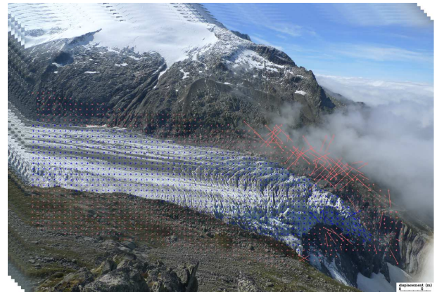
FIGURE 5 – Déplacement en mètre du glacier entre le 19/09/2013 et le 20/09/2013 sur la série droite
