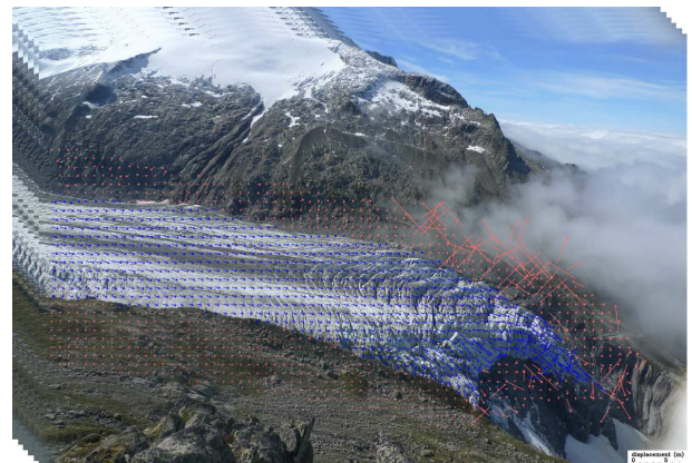
FIGURE 6 – Déplacement en mètre du glacier entre le 19/09/2013 et le 23/09/2013 sur la série droite
