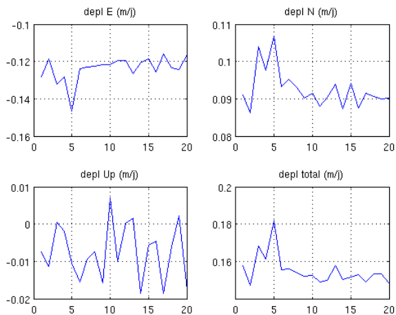
FIGURE 7 – Vitesse en mètre par jour du GéoCube 1006 obtenue par son GPS interne.
