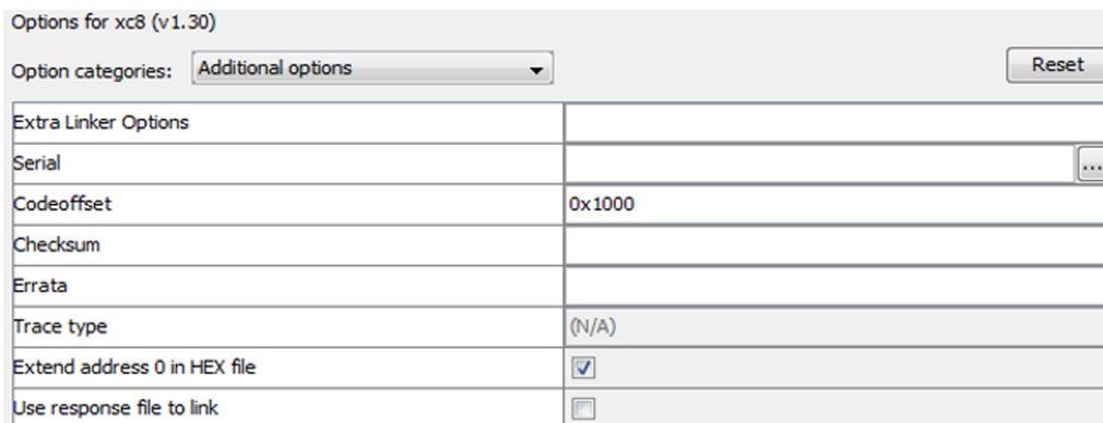
Fig. 3. Se debe especificar al linker de XC8 que la aplicación se cargará a partir de la posición de memoria 0x1000h.
