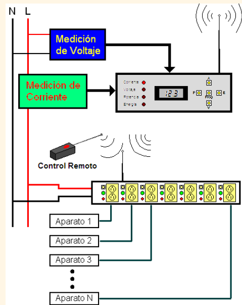
Esquema del monitor visual de consumo de energía eléctrica en viviendas
