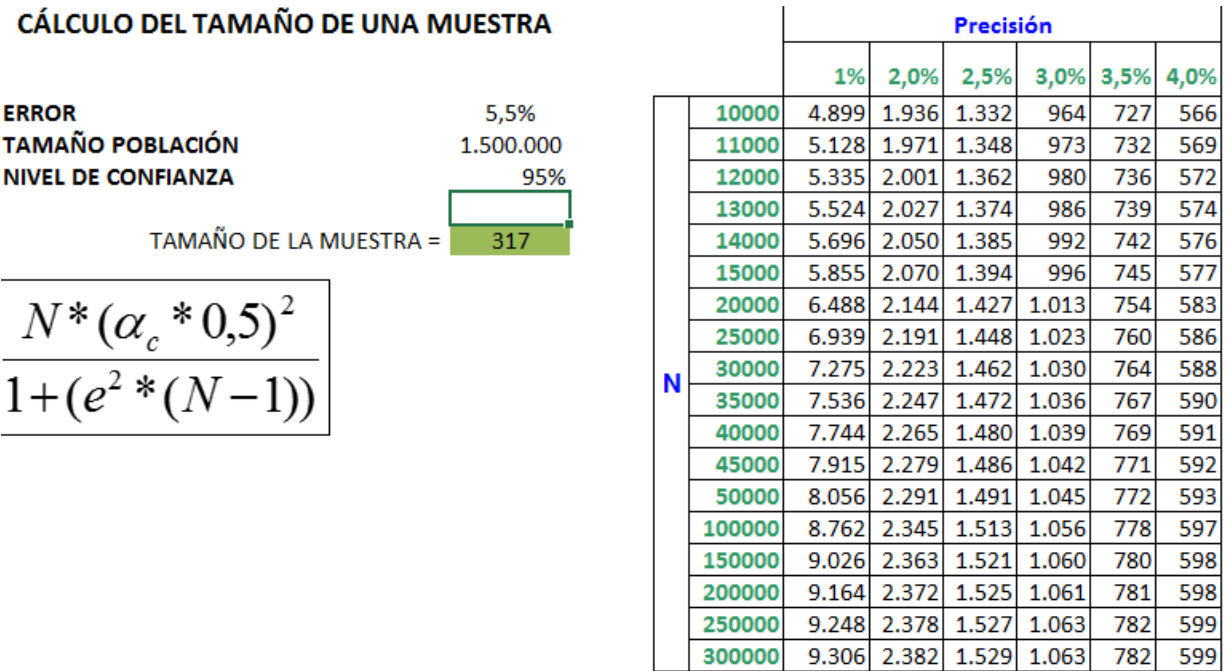
Ilustración 1: Fórmula para cálculo de muestra
