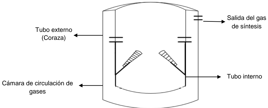
Figura 7. Sección externa del gasificador.
