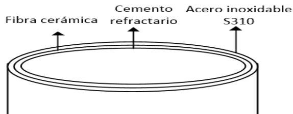
Figura 12. Distribución material tubo interior.
