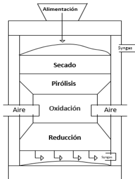
Figura 4. Etapas del proceso de gasificación.
