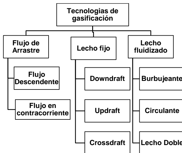
Figura 1. Tipos de gasificadores.
