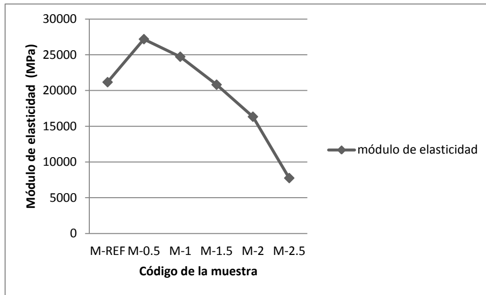
Figura 5.4. Módulo de elasticidad.
