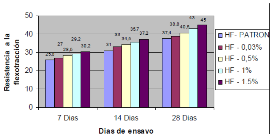
Figura 4.3. Resistencia a la flexotensión [ \text{Kg}/\text{cm}^2 ] (Muñoz, 2007)
