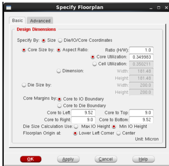
Figure 33. EDI. Floorplan specification
