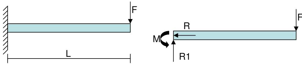
Figura 19. Diagrama de cuerpo libre
