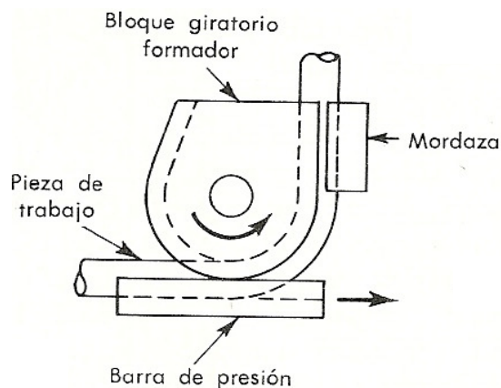
Figura 18. Doblado por estiramiento
