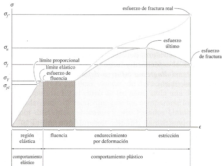
Diagramas esfuerzo-deformación unitaria, convencional y real, para un material dúctil (acero) (no de escala)
