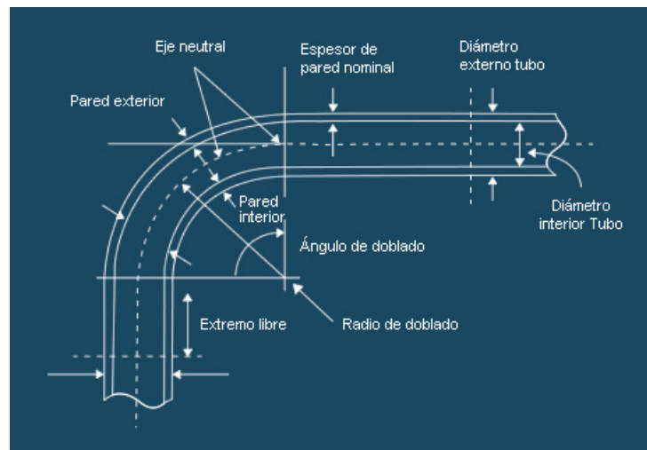
Figura 3. Términos en el doblado de un tubo
