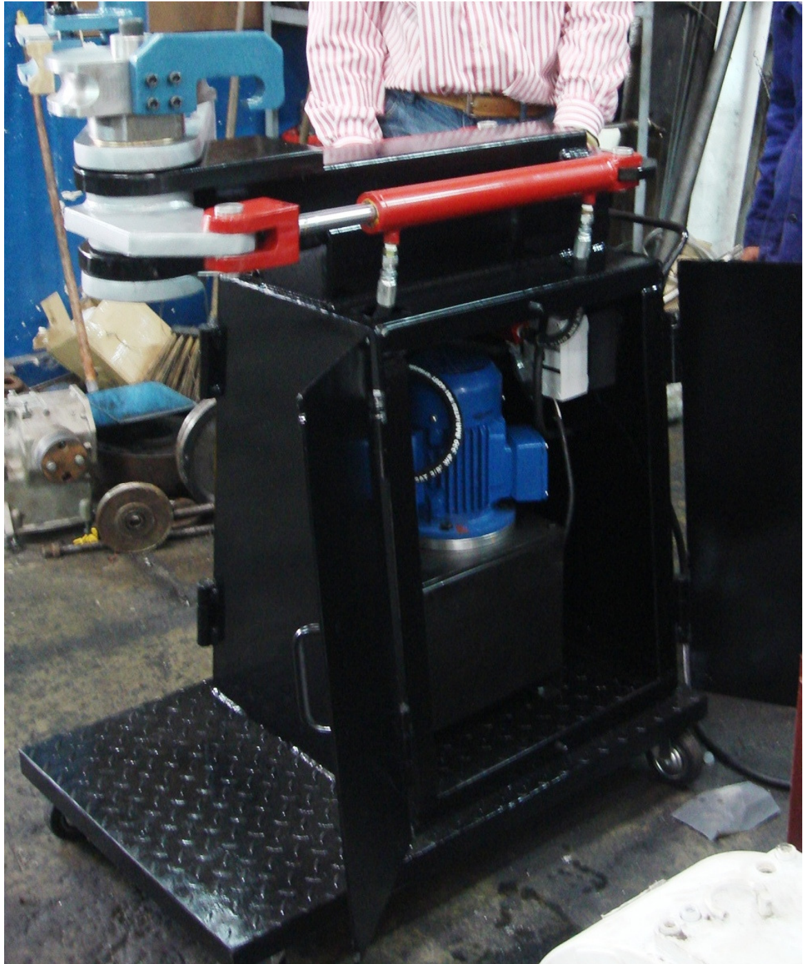
Figura 31. Foto 26: Máquina dobladora totalmente ensamblada vista lateral (prueba de funcionamiento de los cilindros hidráulicos)
