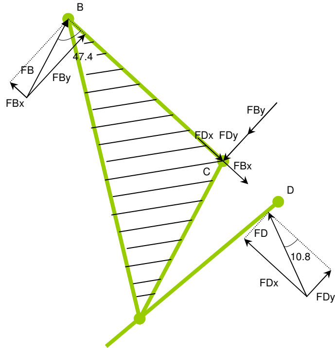
Figura 24. Diagrama de fuerzas del dado formador (barra 4)
