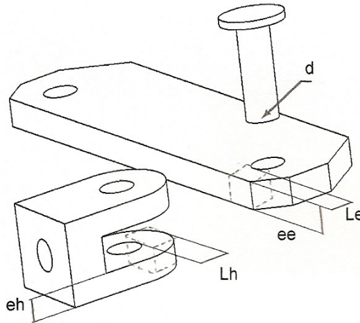
Figura 27. Horquillas, eslabón y pasador
