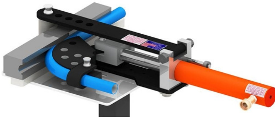
Figura 14. Dobladora hidráulica Pro-tools HB 302 - 15 Ton
