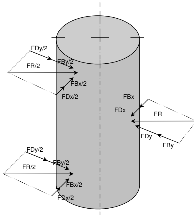
Figura 25. Esfuerzos cortantes en el eje principal
