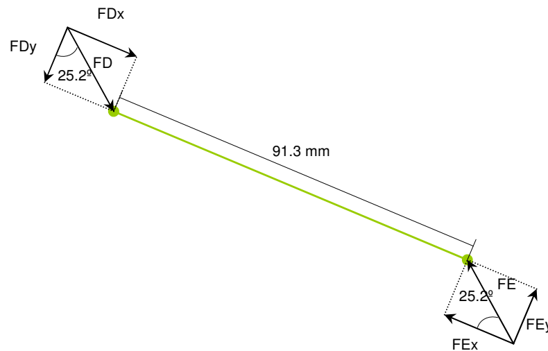
Figura 23. Diagrama de fuerzas de la barra 6
