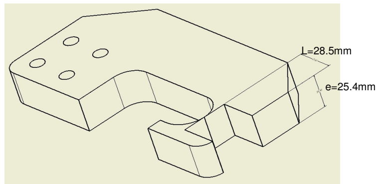
Figura 28. Sujetador del tubo en C
