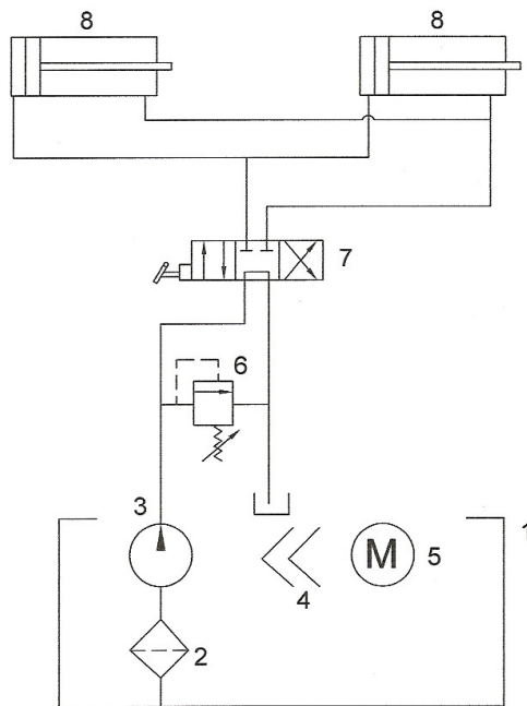
Figura 29. Plano hidráulico
