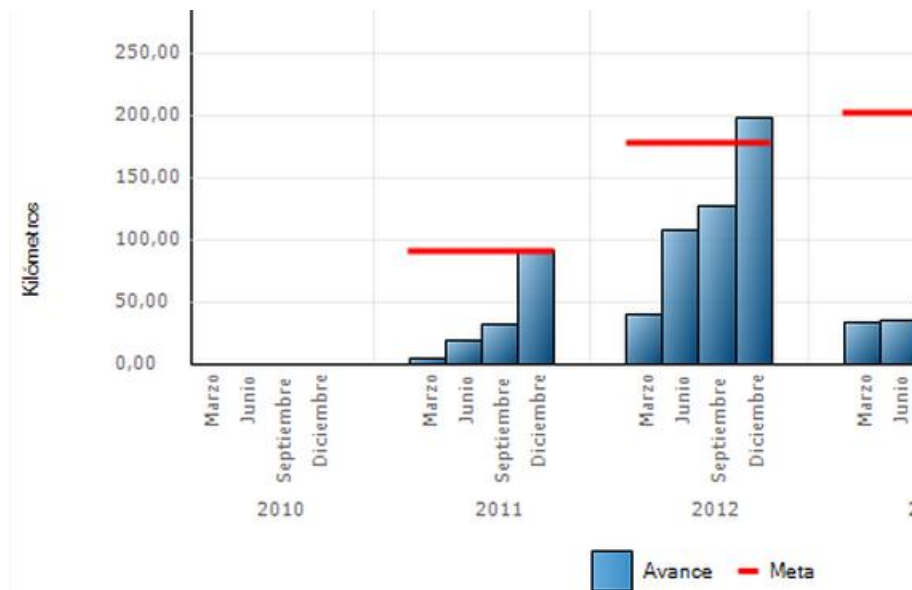
Imágen 10. Avance en kilómetros de doble calzada en operación
