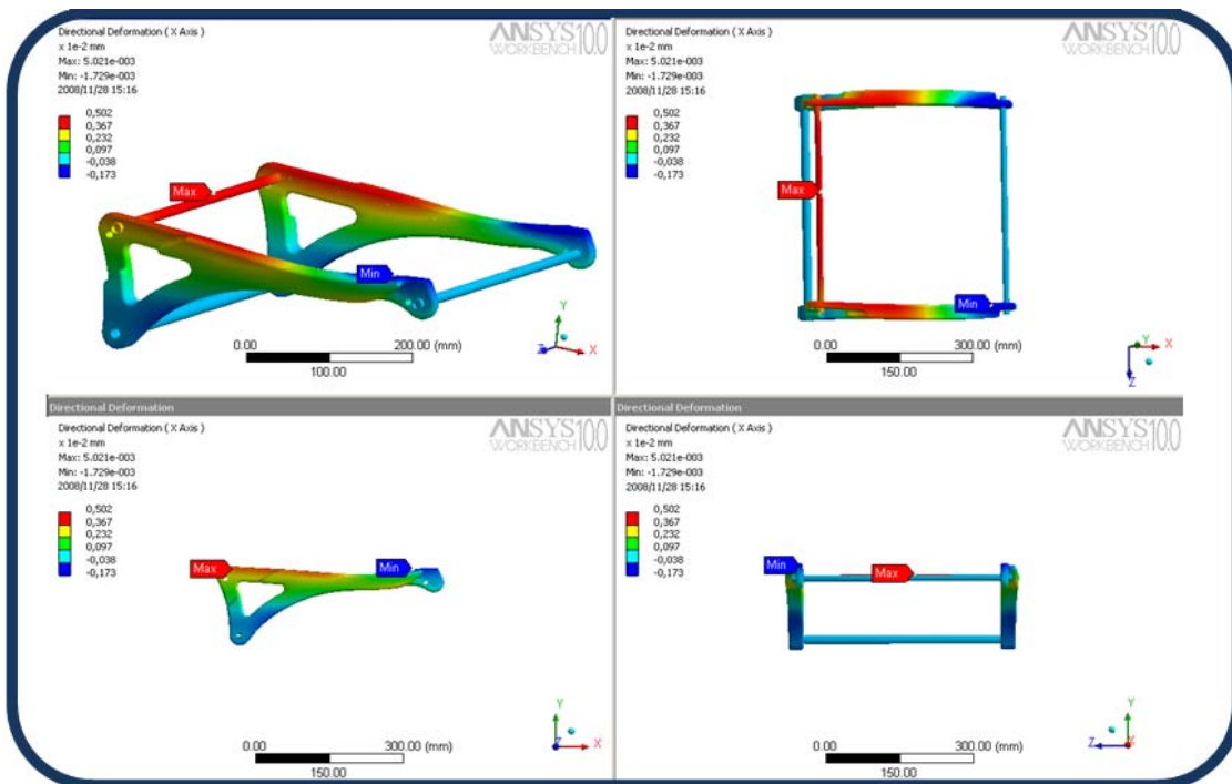
Imagen 22: Deformación máxima sobre la estructura ampliada 1000 veces
