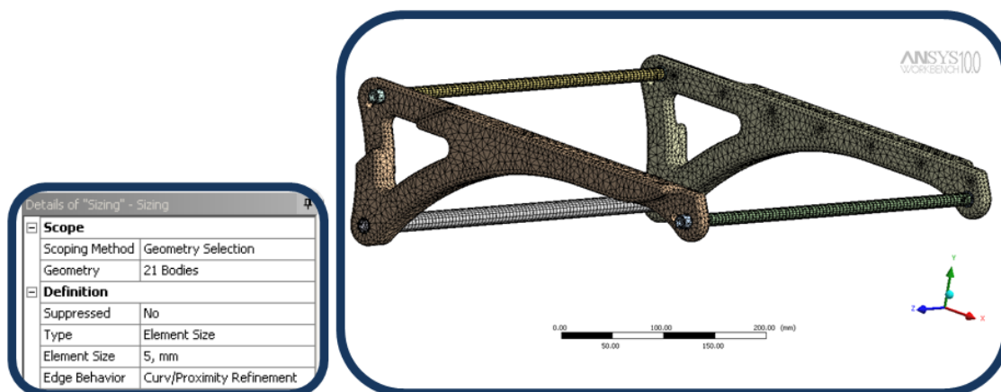
Imagen 19: Mallado de la pieza
