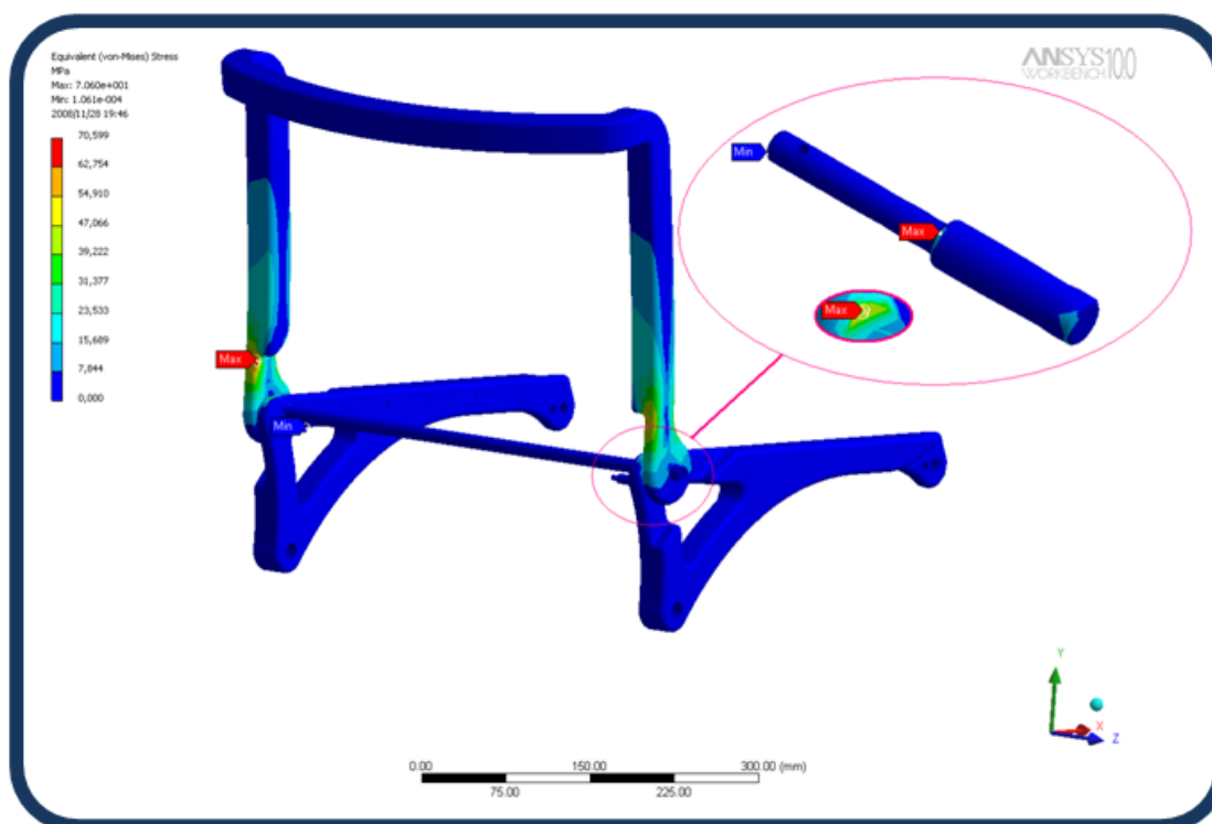
Imagen 24: Esfuerzos máximos sobre el espaldar y sus respectivos seguros
