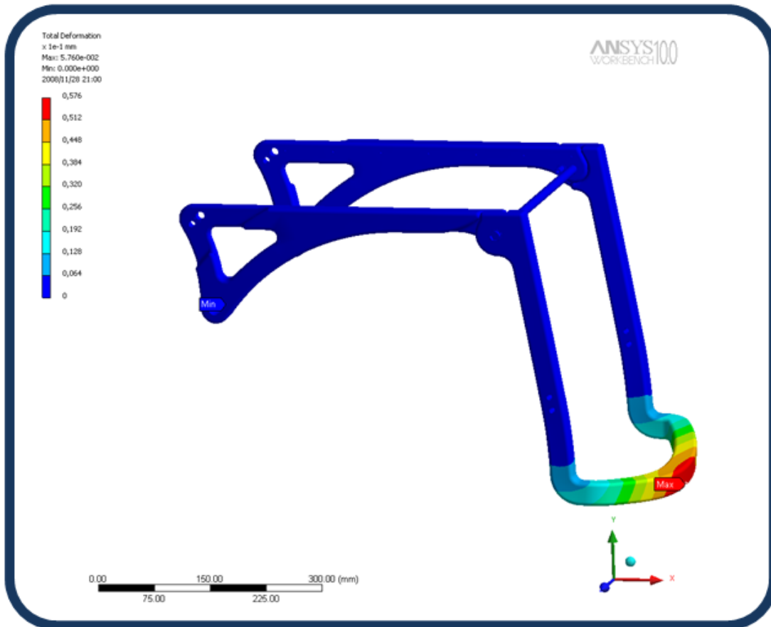
Imagen 27: Deformación máxima sobre el apoya pies ampliada 1000 veces
