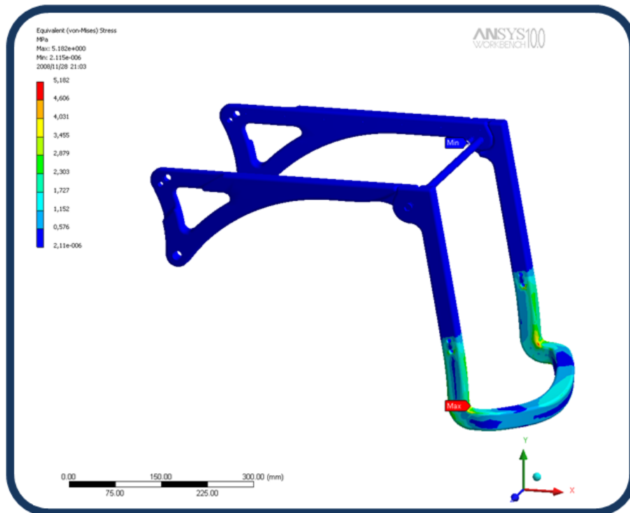
Imagen 26: Esfuerzos máximos sobre el apoya pies y sus seguros
