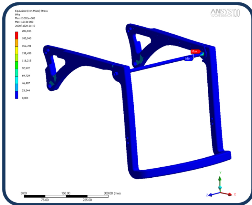
Imagen 29: Esfuerzos máximos en bujes y seguros
