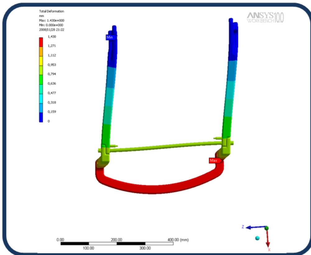
Imagen 30: Deformaciones máximas sobre reposa pies, bujes, tornillos y seguros escala x 1000
