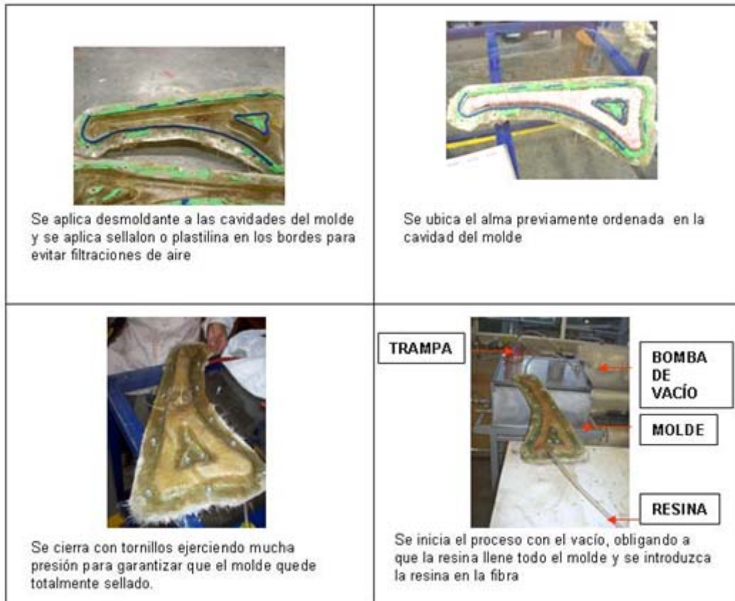
Imagen 43: Prueba inyección por VM
