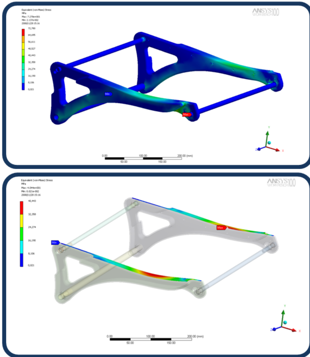
Imagen 21: Deformación del chasis ampliada 1000 veces
