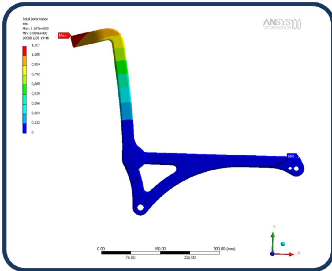
Imagen 25: Deformación máxima sobre el espaldar ampliada 1000 veces
