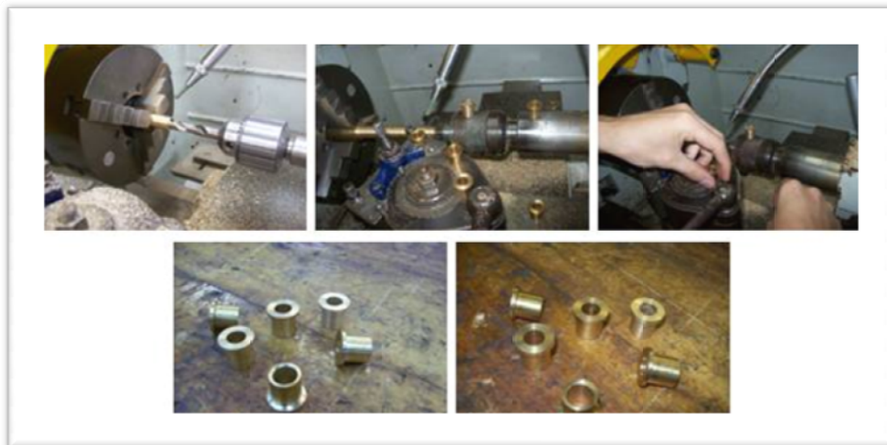
Imagen 34: Elaboración de bujes
