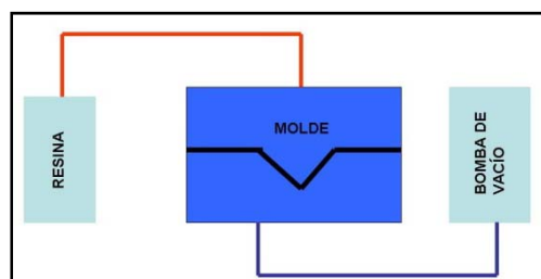
Imagen 40: Sistema de proceso VM
