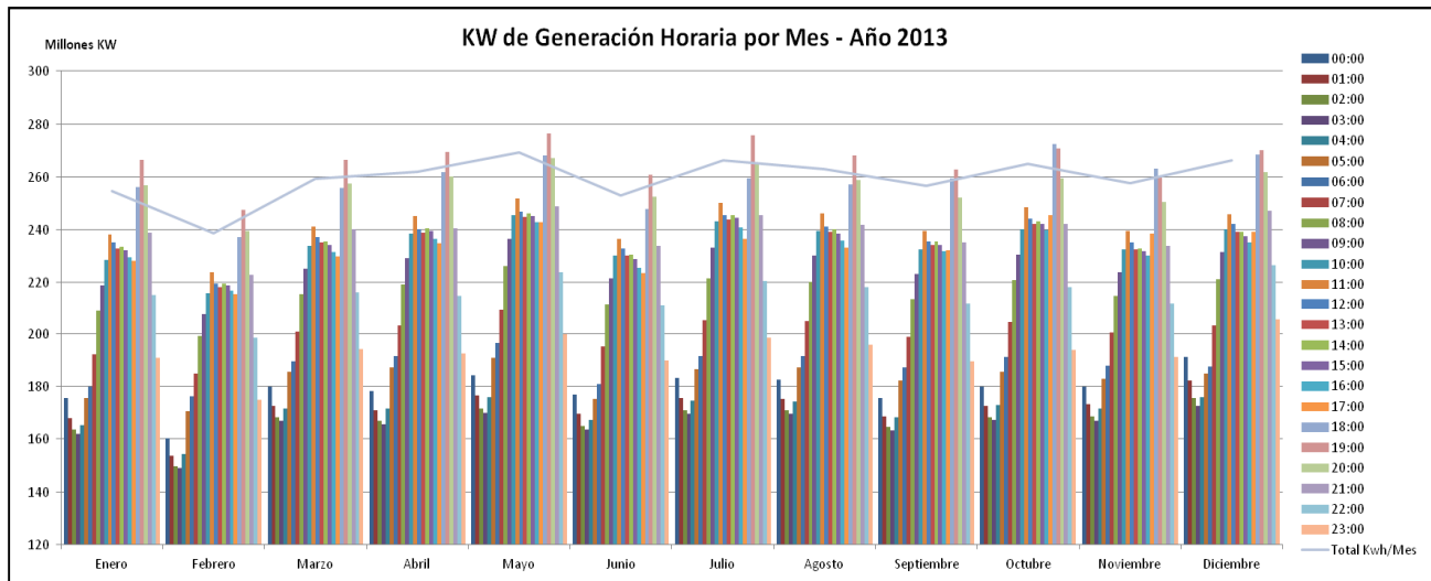
Gráfico 6. Generación Horaria por Mes - 2013
