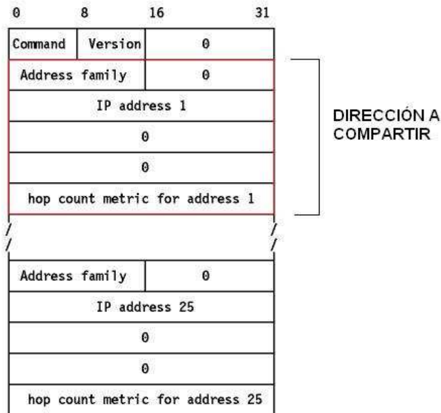
Figura 10.8: Encapsulamiento de registro en mensaje de respuesta RIP. Fuente: RFC 1058.
