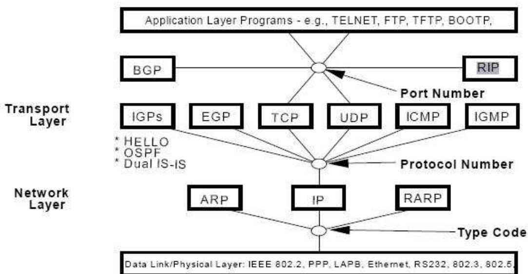
Figura 10.5: Familia de protocolos TCP/IP
