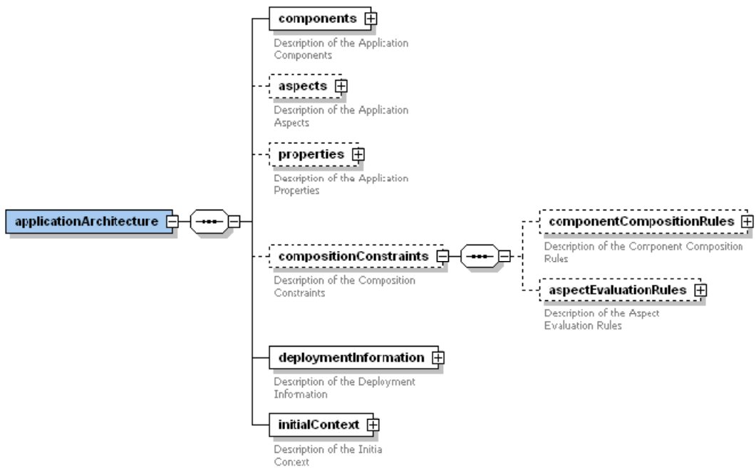
Figura 8. Estructura del lenguaje DAOP-ADL Fuente: [2]
