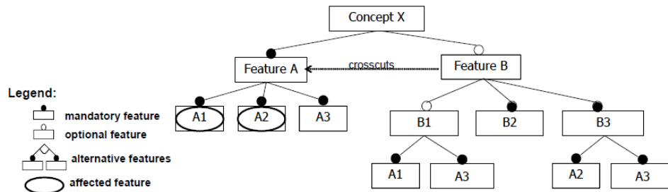
Figura 10. Crosscutting feature models Fuente: [2]
