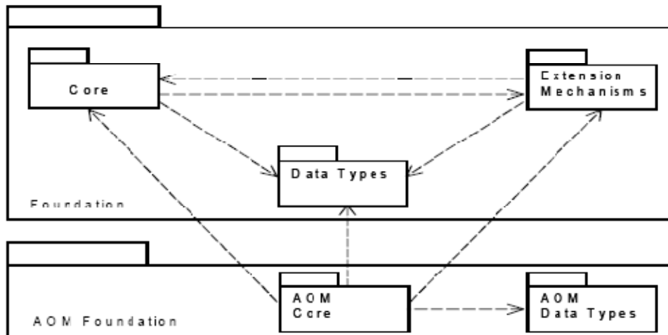
Figura 6. Vista de paquete de alto nivel del espacio UML para AOM
