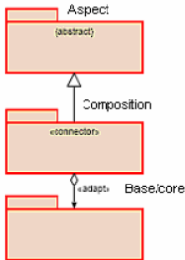
Figura 16. Nivel de Composición de un Paquete Fuente: [2]
