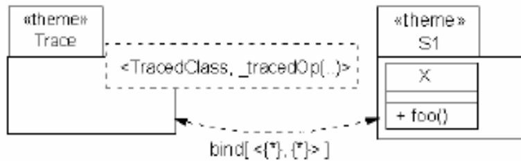
Figura 14. Themes e integración de Themes
