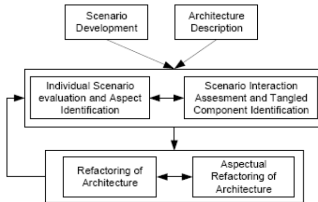
Figura 12. Actividades de ASAAM Fuente: [2]
